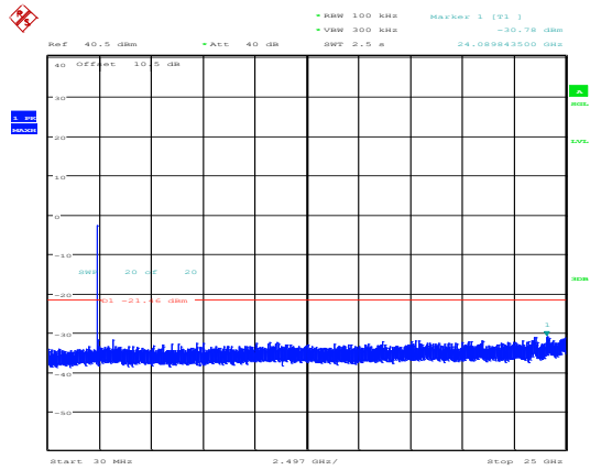
802.11n20_2412MHz_Chain 1
