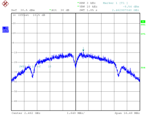
802.11b_2462MHz_Chain 0
