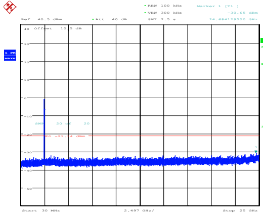
802.11n20_2462MHz_Chain 1
