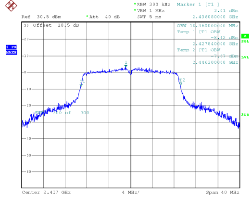
802.11n20_2437MHz_Chain 0
