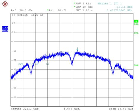
802.11b_2412MHz_Chain 0
