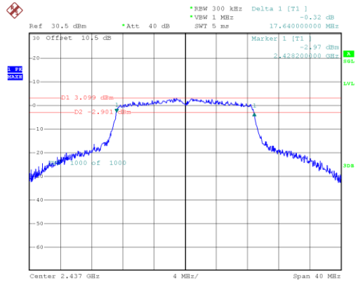
802.11n20_2437MHz_Chain 0
