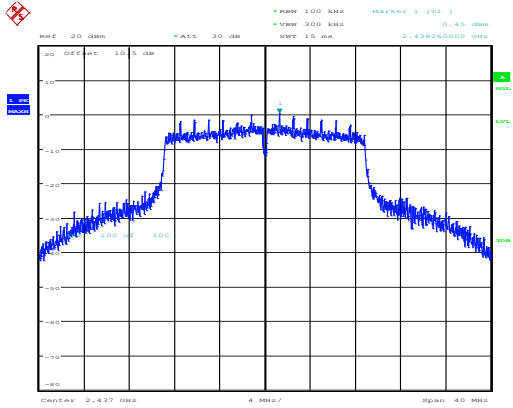
802.11n20_2437MHz_Chain 0
