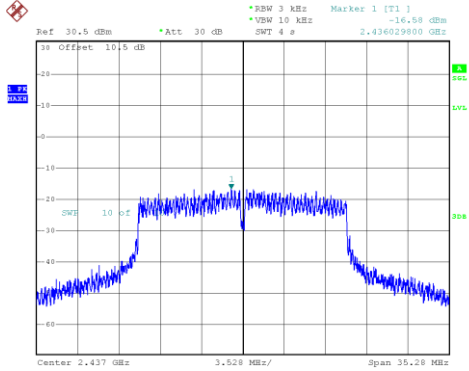
802.11n20_2437MHz_Chain 1
