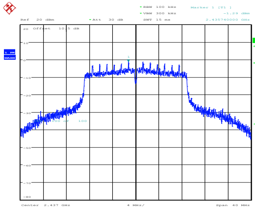
802.11n20_2437MHz_Chain 1
