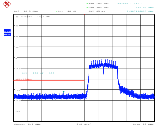
802.11n20_2412MHz_Chain 1
