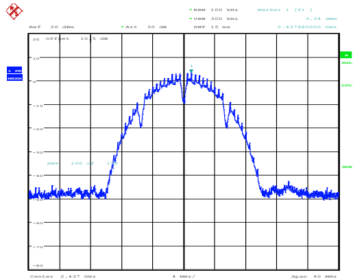
802.11b_2437MHz_Chain 1
