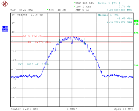
802.11b_2412MHz_Chain 0
