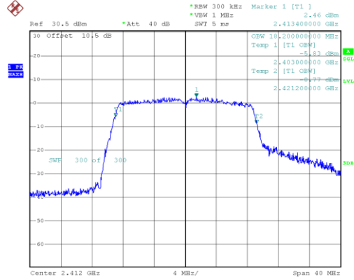
802.11n20_2412MHz_Chain 0
