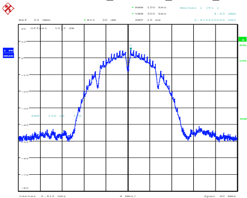
802.11b_2412MHz_Chain 0_
