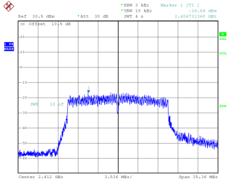
802.11n20_2412MHz_Chain 1
