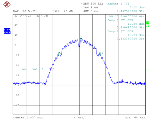
802.11b_2437MHz_Chain 0
