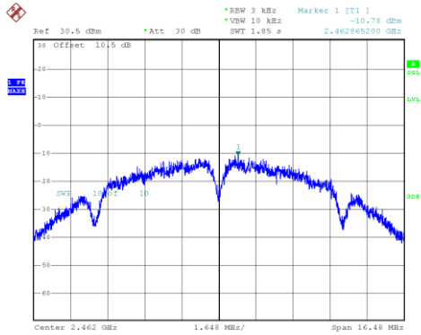
802.11b_2462MHz_Chain 1
