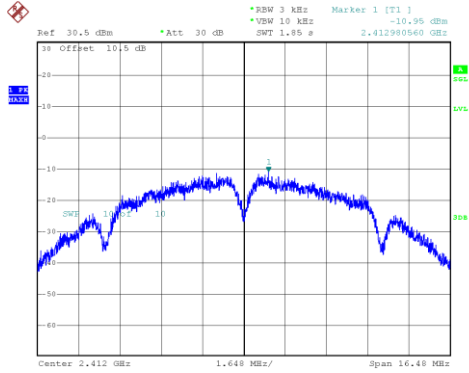
802.11b_2412MHz_Chain 1
