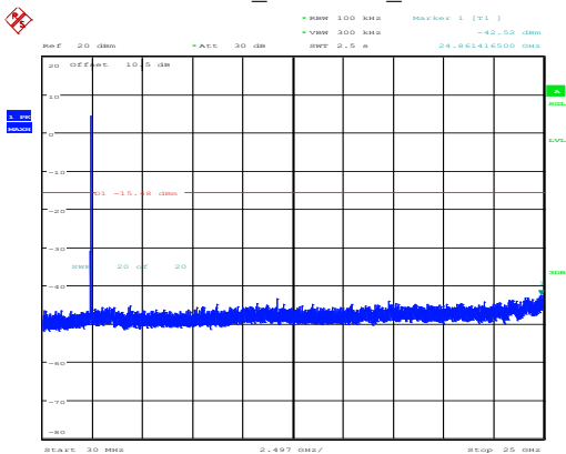
802.11b_2437MHz_Chain 0
