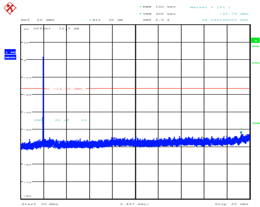
802.11b_2437MHz_Chain 1
