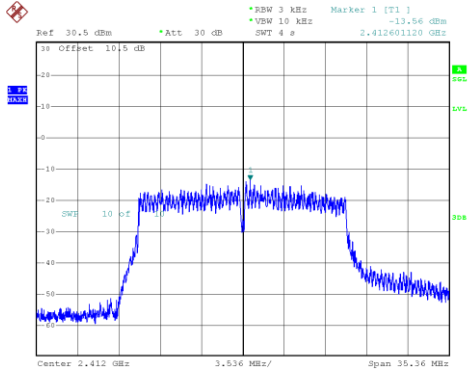
802.11n20_2412MHz_Chain 0
