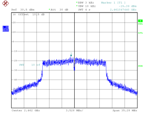
802.11n20_2462MHz_Chain 1
