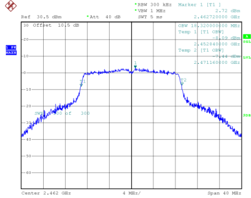
802.11n20_2462MHz_Chain 0
