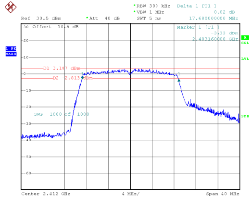
802.11n20_2412MHz_Chain 0
