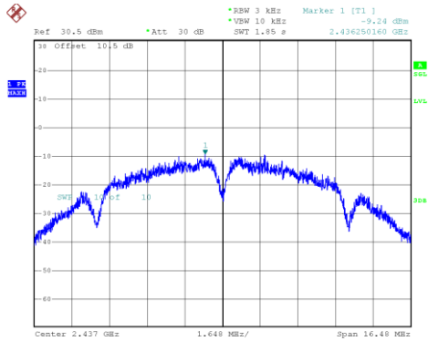
802.11b_2437MHz_Chain 0
