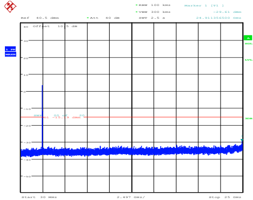
802.11b_2462MHz_Chain 0
