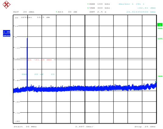
802.11n20_2437MHz_Chain 1
