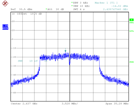
802.11n20_2437MHz_Chain 0
