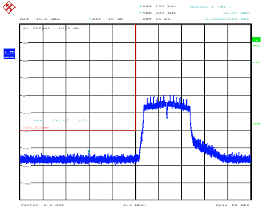
802.11n20_2412MHz_Chain 0
