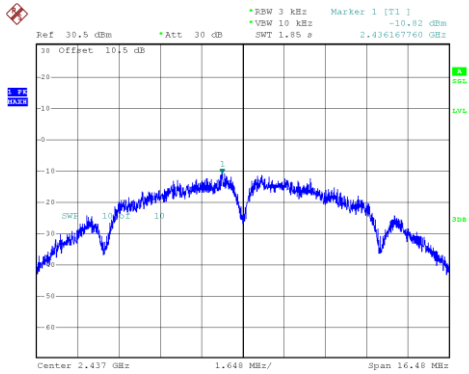
802.11b_2437MHz_Chain 1
