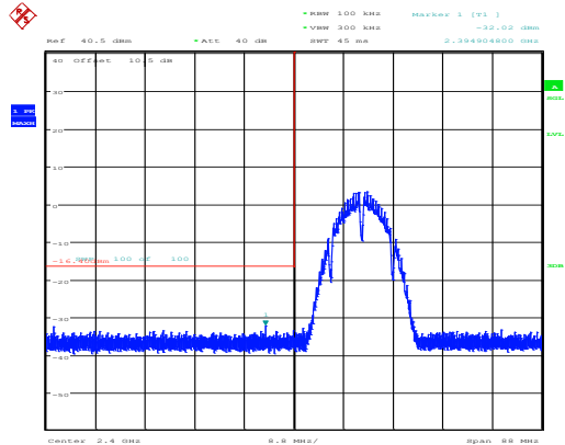
802.11b_2412MHz_Chain 1
