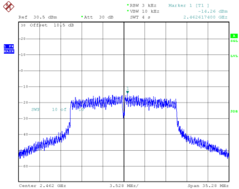
802.11n20_2462MHz_Chain 0
