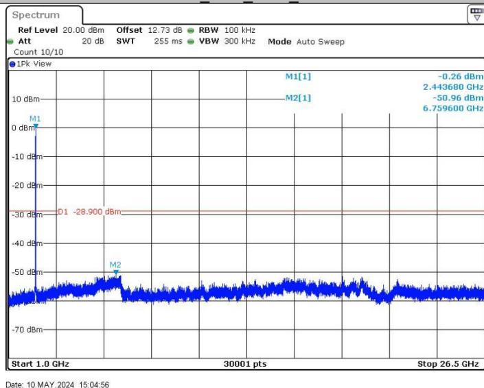
11AX20SISO_Ant2_2437_1000~26500
