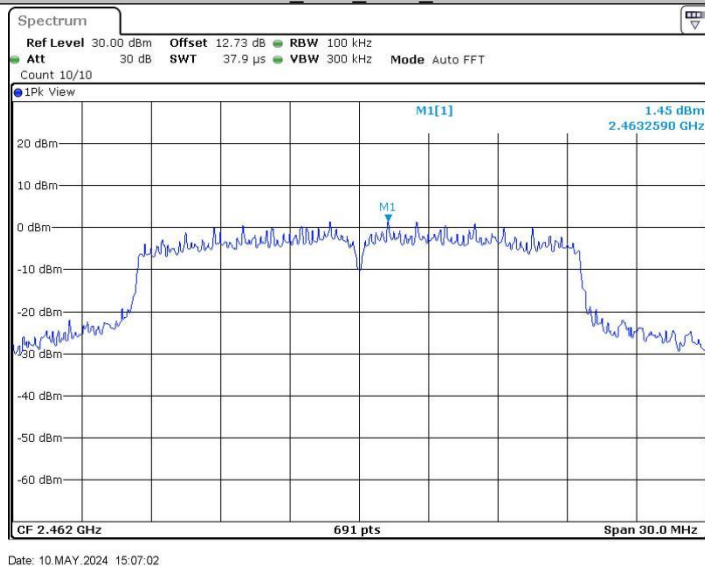
11AX20SISO_Ant2_2462_0~Reference
