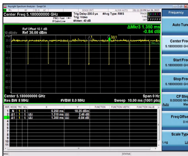
802.11ac VHT20
