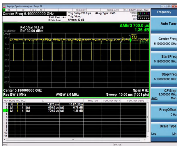
802.11ac VHT40
