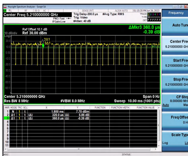
802.11ac VHT80
