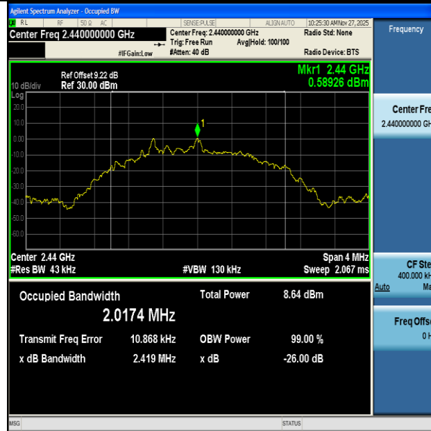
BLE_2M-Ant1-2440
