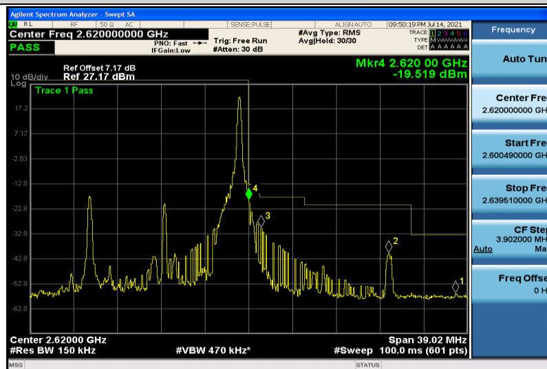
Band38-15MHz-QPSK-38175-1RB#74
