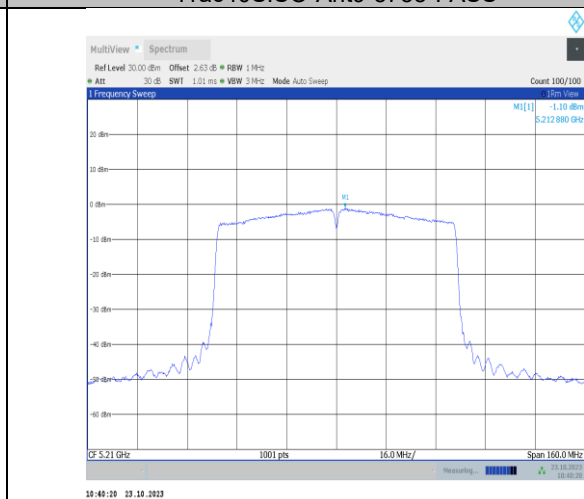
11ac80SISO-Ant9-5210-PASS
