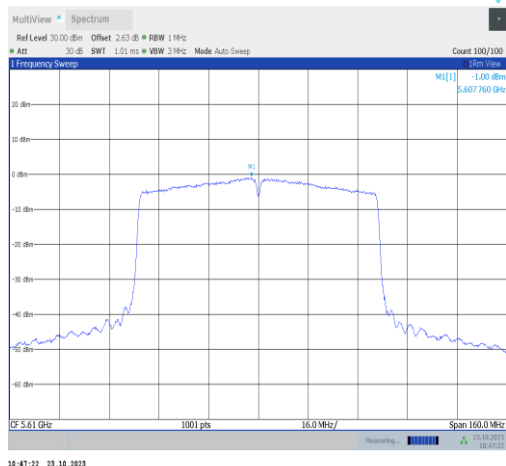
11ac80SISO-Ant9-5610-PASS
