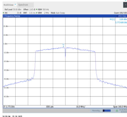
11ac80SISO-Ant9-5775-PASS
