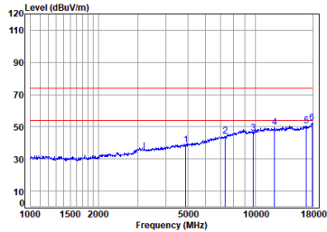
11n_40M_TX_CH_09_Horizontal
