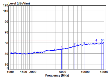
11n_40M_TX_CH_06_Horizontal
