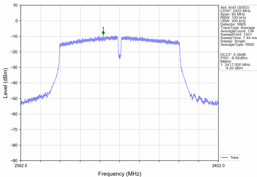
802.11n(HT40)_LCH_2422MHz_Ant3 (SISO)_NTNV
