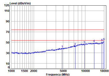
11n_40M_TX_CH_06_Vertical
