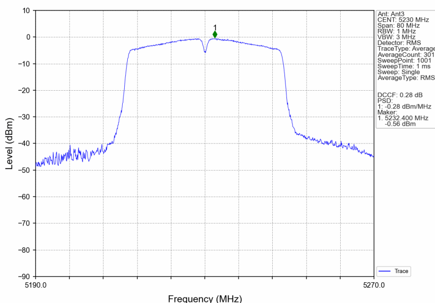
802.11n(HT40)_HCH_5230MHz_Ant3_NTNV
