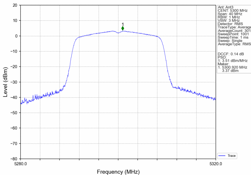
802.11n(HT20)_MCH_5300MHz_Ant3_NTNV
