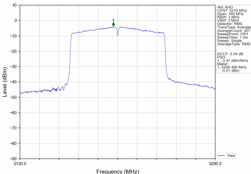
802.11ac(VHT80)_MCH_5210MHz_Ant3_NTNV
