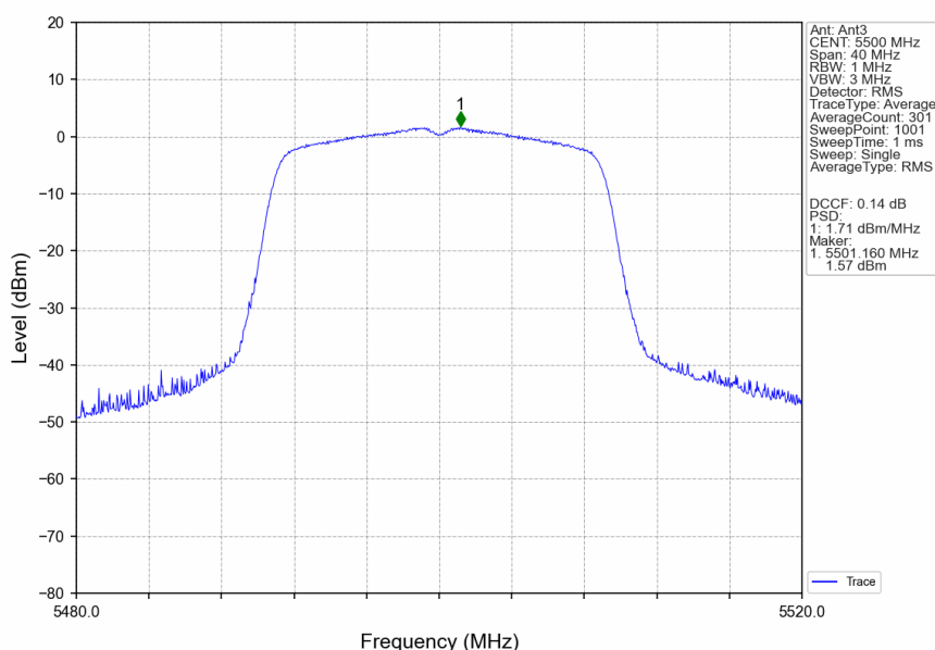
802.11n(HT20)_LCH_5500MHz_Ant3_NTNV
