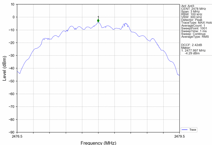
2M_HCH_2478MHz_Ant3_NTNV
