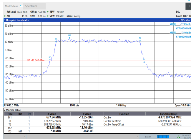
Band71-5MHz-QPSK-133297-25RB#0
