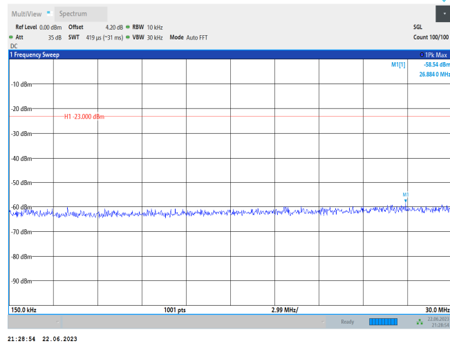
Band2-20MHz-QPSK-18700-1RB#0-Range2:0.15~30MHz
