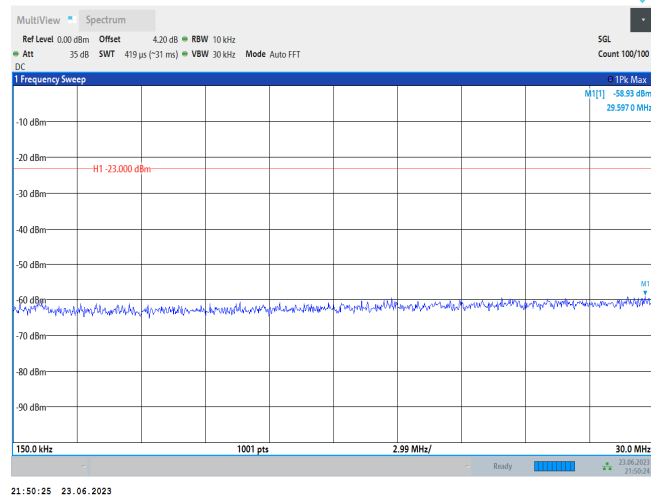
Band12-10MHz-QPSK-23060-1RB#0-Range2:0.15~30MHz
