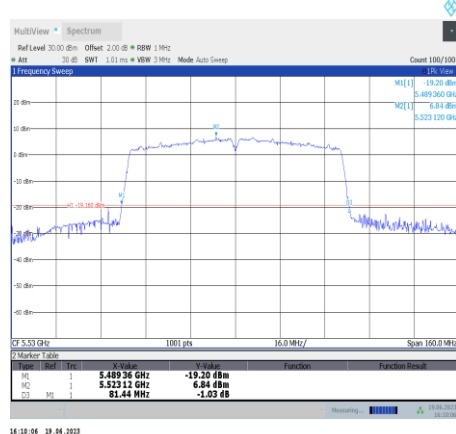
11ac80SISO-Ant11-5530
