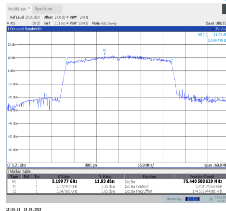
11ac80SISO-Ant11-5210
