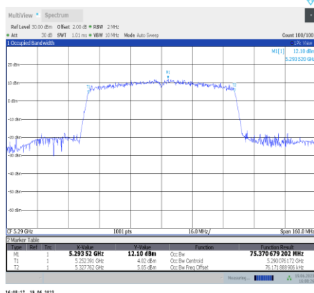
11ac80SISO-Ant11-5290
