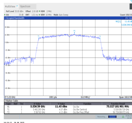
11ac80SISO-Ant11-5530
