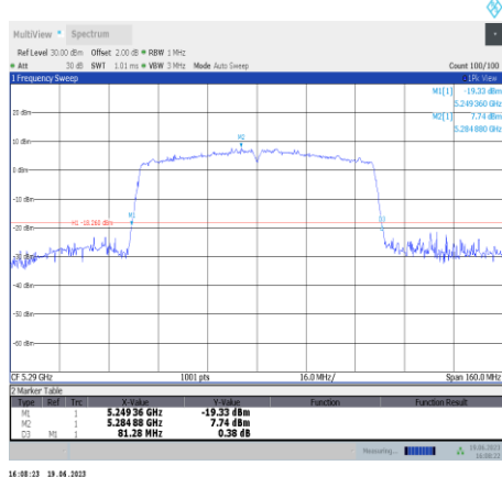
11ac80SISO-Ant11-5290
