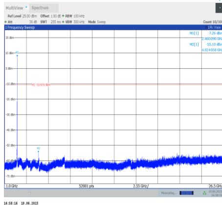
11b-Ant9-2462-1000~26500
