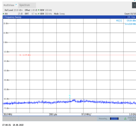
11g-Ant9-2412-30~1000
