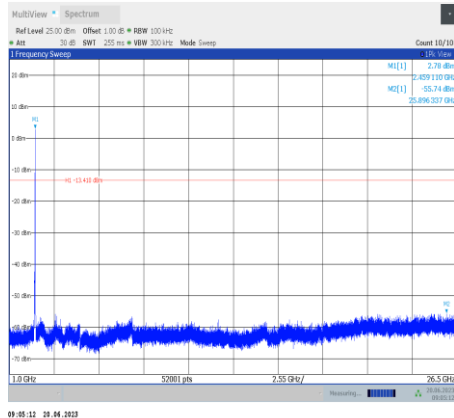
11n20SISO-Ant9-2462-1000~26500
