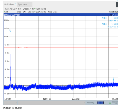
11g-Ant9-2412-1000~26500
