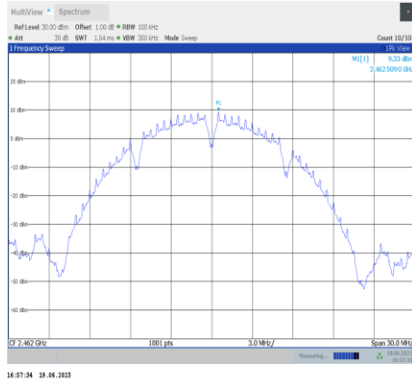
11b-Ant9-2462-0~Reference
