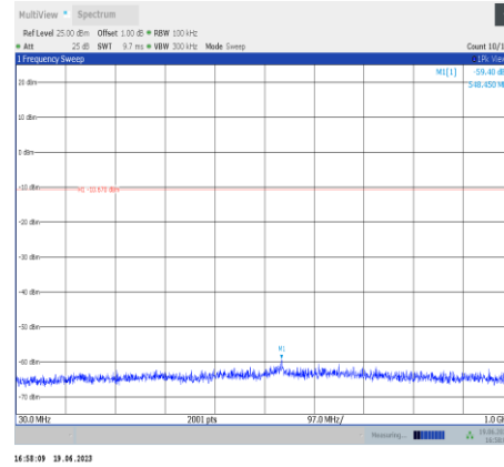
11b-Ant9-2462-30~1000
