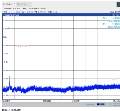
11b-Ant9-2412-1000~26500
