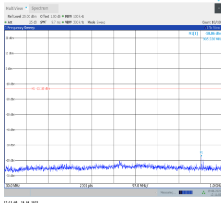
11g-Ant9-2462-30~1000
