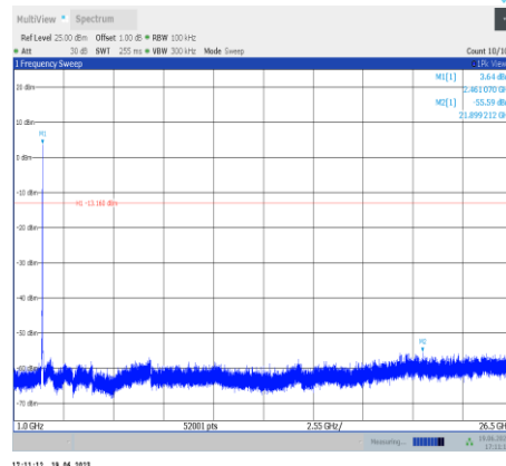
11g-Ant9-2462-1000~26500
