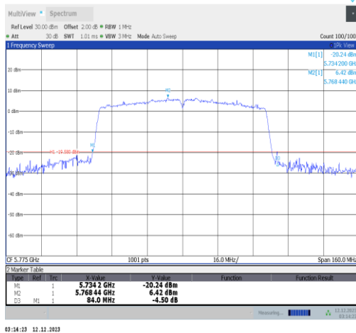
11ac80SISO-Ant2-5775
