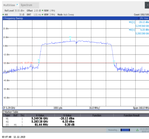
11ac80SISO-Ant2-5290
