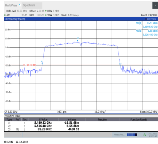
11ac80SISO-Ant2-5530
