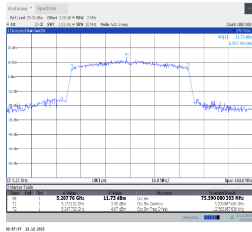
11ac80SISO-Ant2-5210
