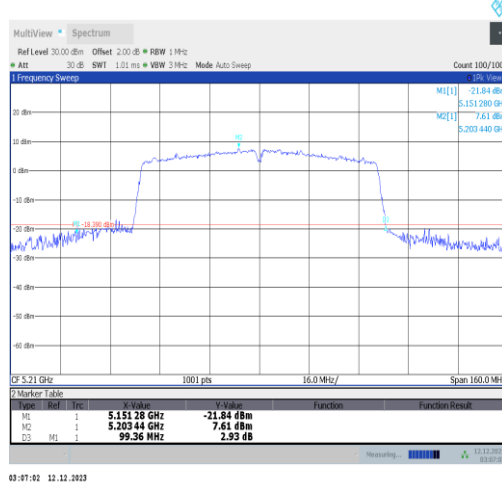
11ac80SISO-Ant2-5210
