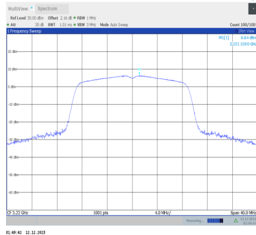
11n20ISO-Ant2-5220-PASS
