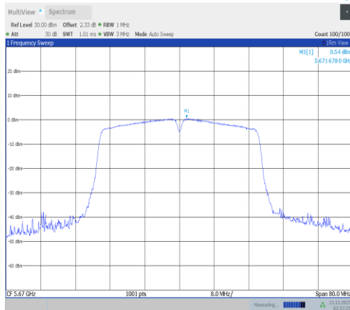
11n40ISO-Ant2-5670-PASS
