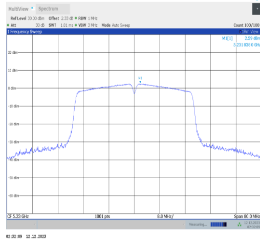
11n40ISO-Ant2-5230-PASS
