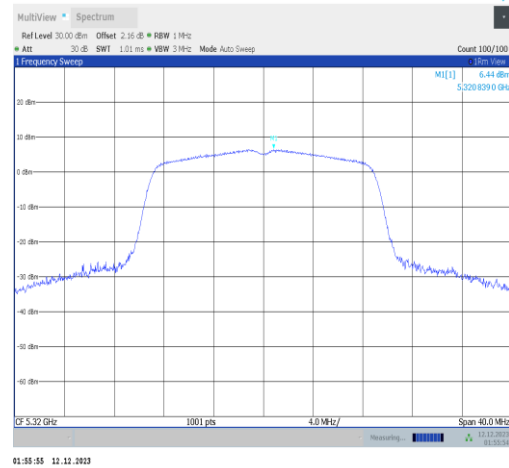
11n20ISO-Ant2-5320-PASS
