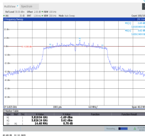
11n20ISO-Ant2-5825-PASS
