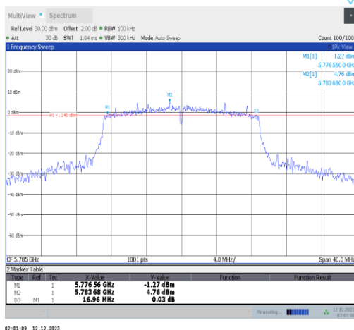
11n20ISO-Ant2-5785-PASS
