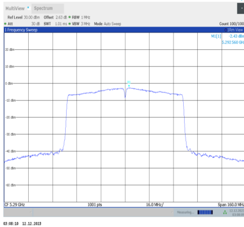
11ac80SISO-Ant2-5290-PASS
