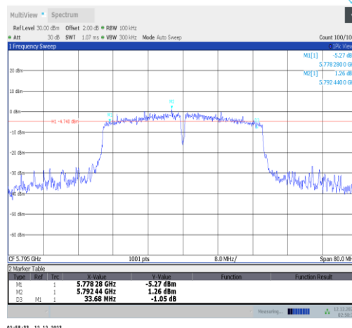
11n40ISO-Ant2-5795-PASS
