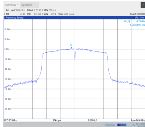
11n40ISO-Ant2-5755-PASS
