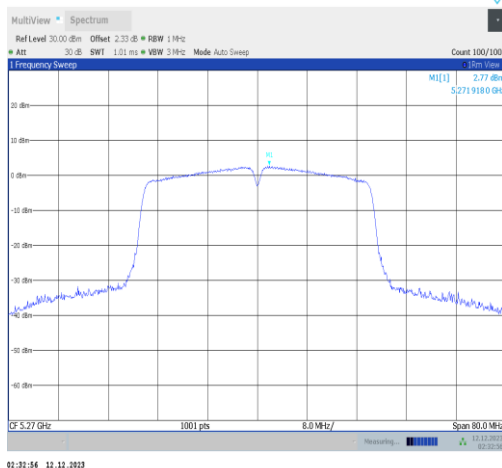
11n40ISO-Ant2-5270-PASS
