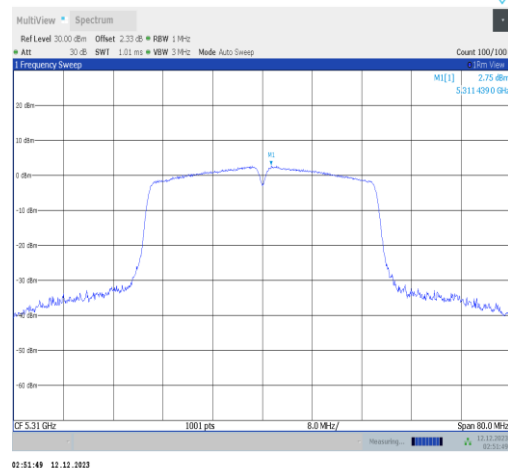
11n40ISO-Ant2-5310-PASS
