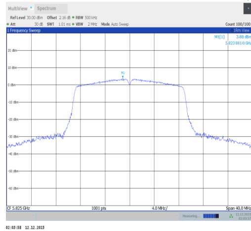
11n20ISO-Ant2-5825-PASS
