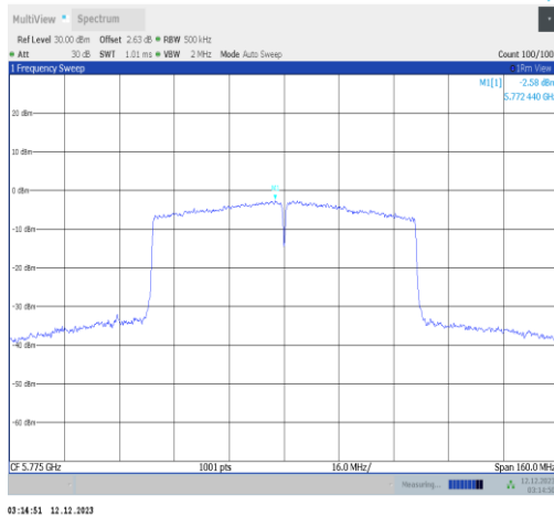
11ac80SISO-Ant2-5775-PASS
