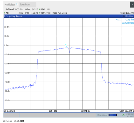
11ac80SISO-Ant2-5530-PASS
