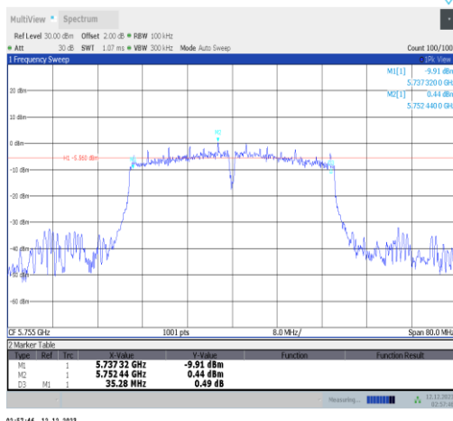
11n40ISO-Ant2-5755-PASS
