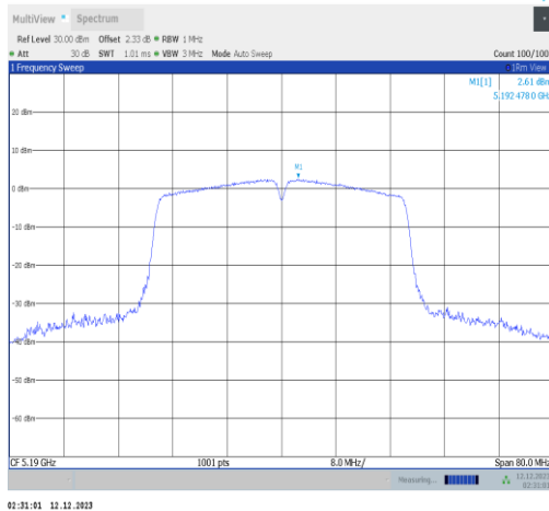
11n40ISO-Ant2-5190-PASS
