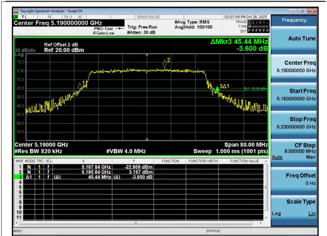
11AX40MIMO-Ant1-5190
