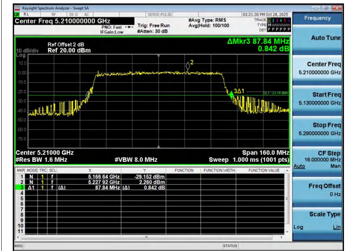
11AX80MIMO-Ant2-5210
