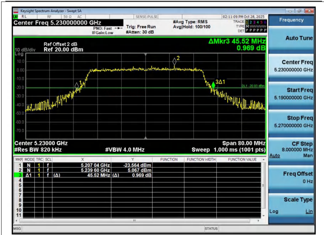
11AX40MIMO-Ant1-5230
