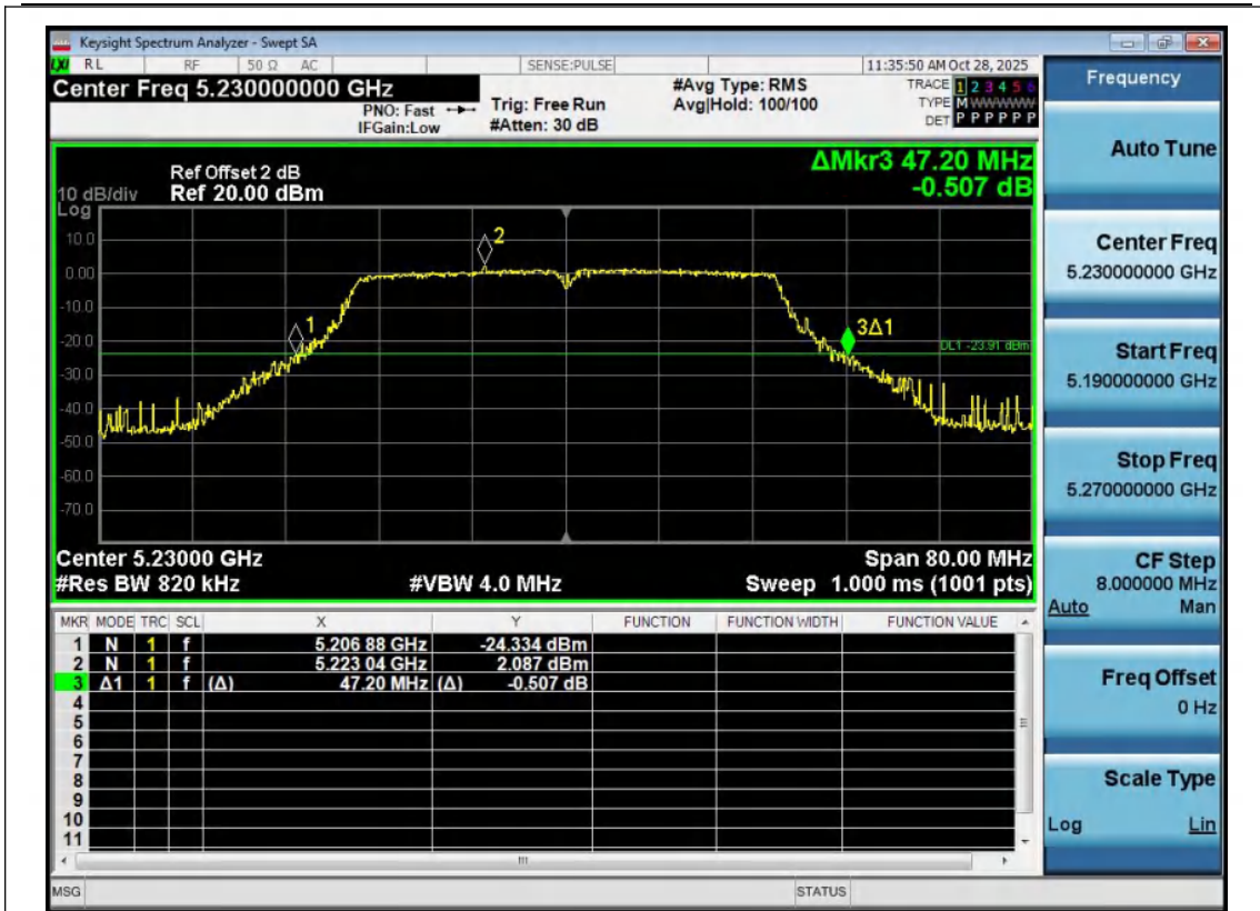
11AC40MIMO-Ant1-5230
