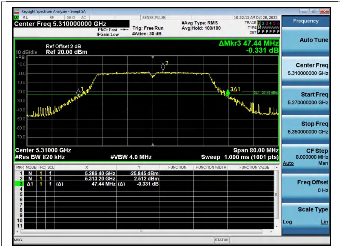
11N40MIMO-Ant1-5310
