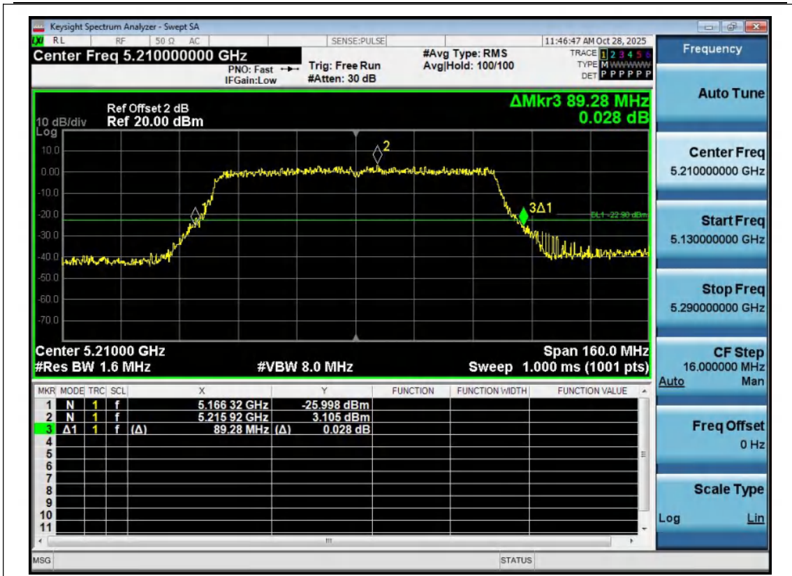
11AC80MIMO-Ant1-5210
