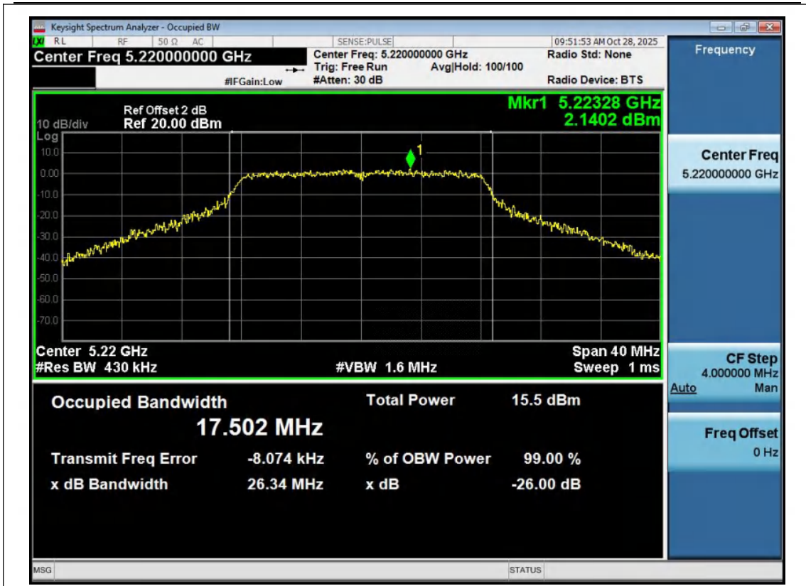
11A-Ant1-5220
