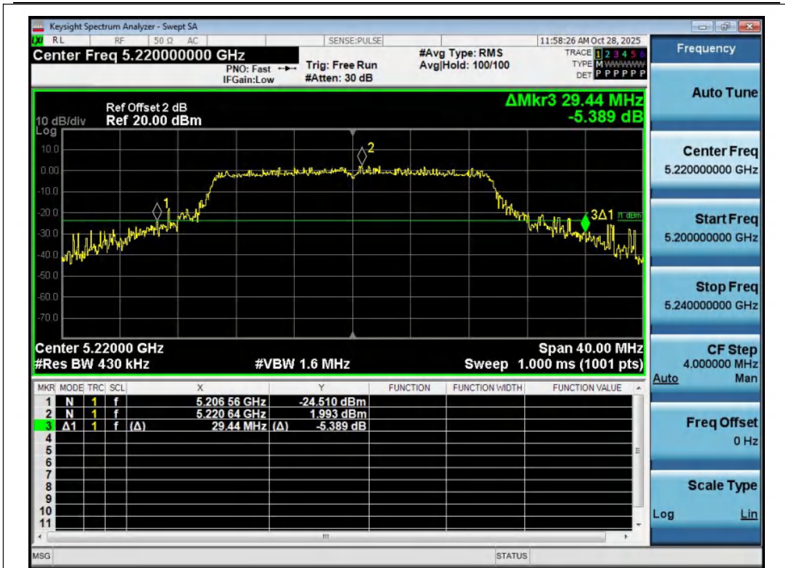
11AX20MIMO-Ant1-5220
