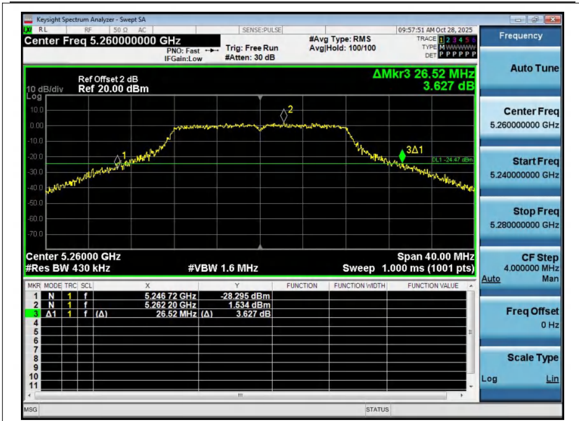
11A-Ant1-5260
