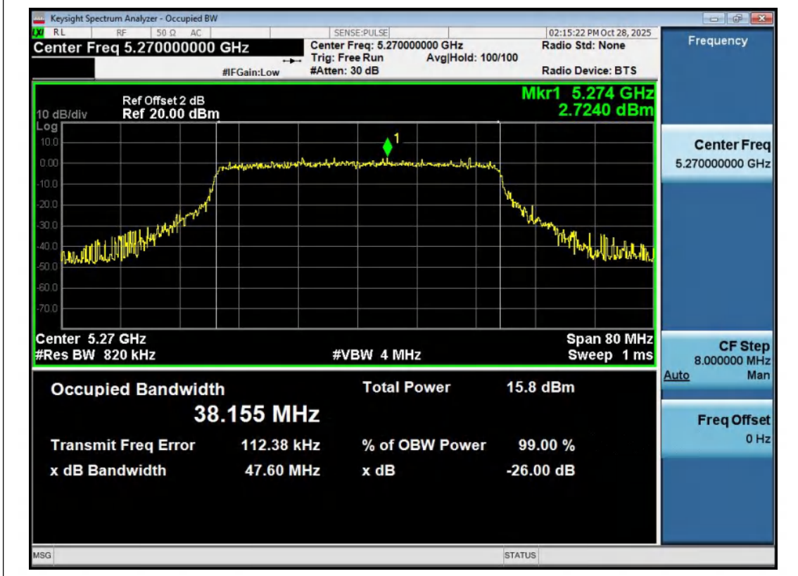
11AX40MIMO-Ant2-5270
