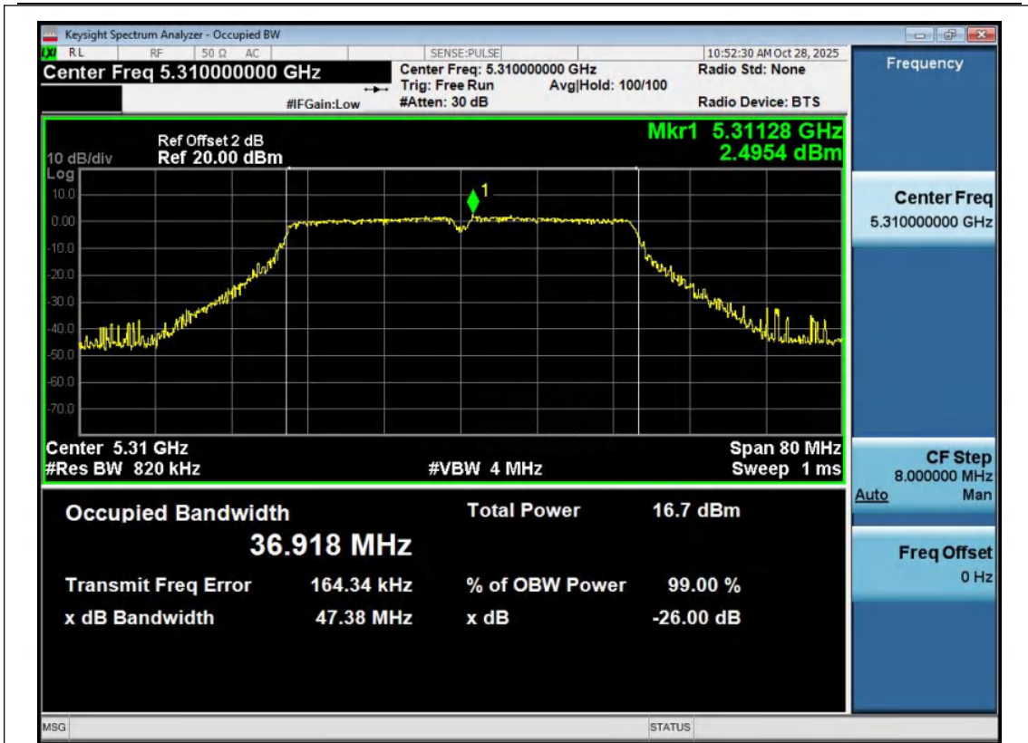
11N40MIMO-Ant1-5310
