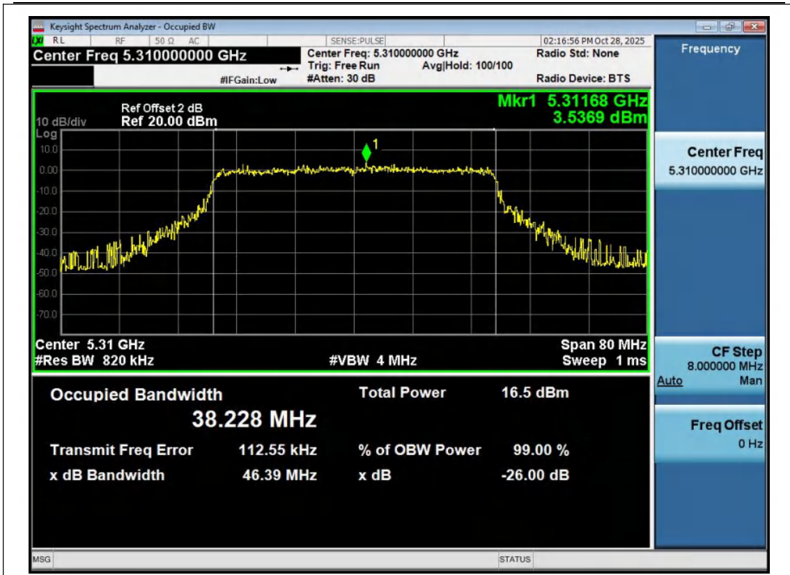
11AX40MIMO-Ant1-5310
