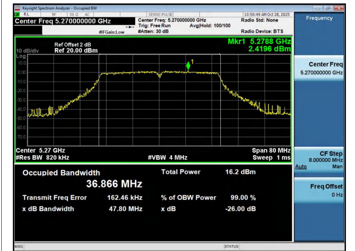
11N40MIMO-Ant2-5270
