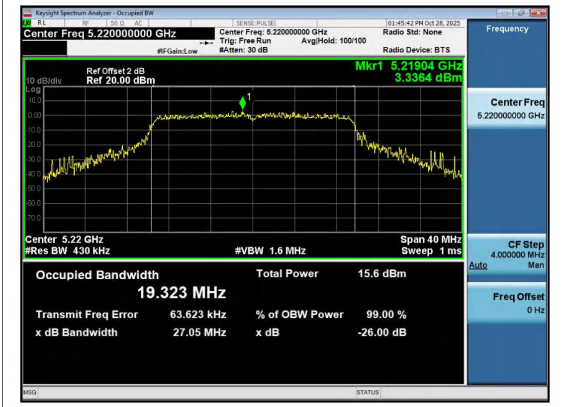
11AX20MIMO-Ant2-5220
