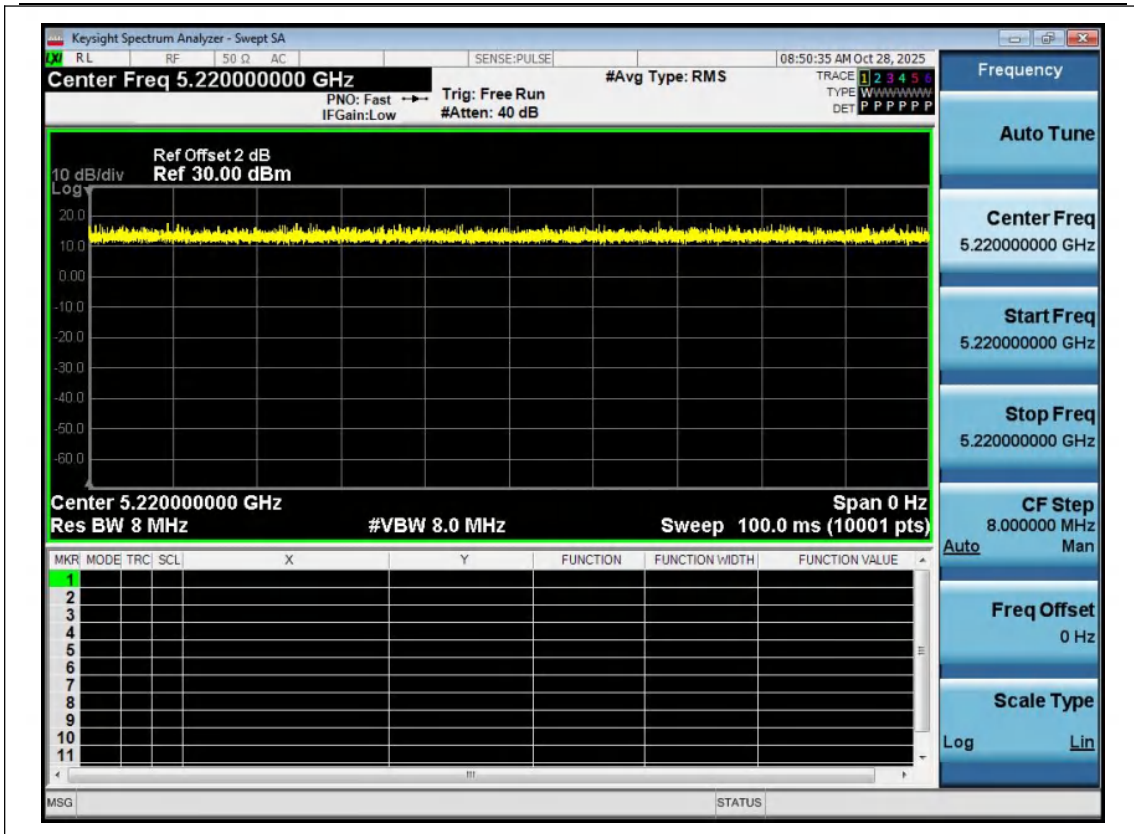
NTNV-11A-Ant1-5220
