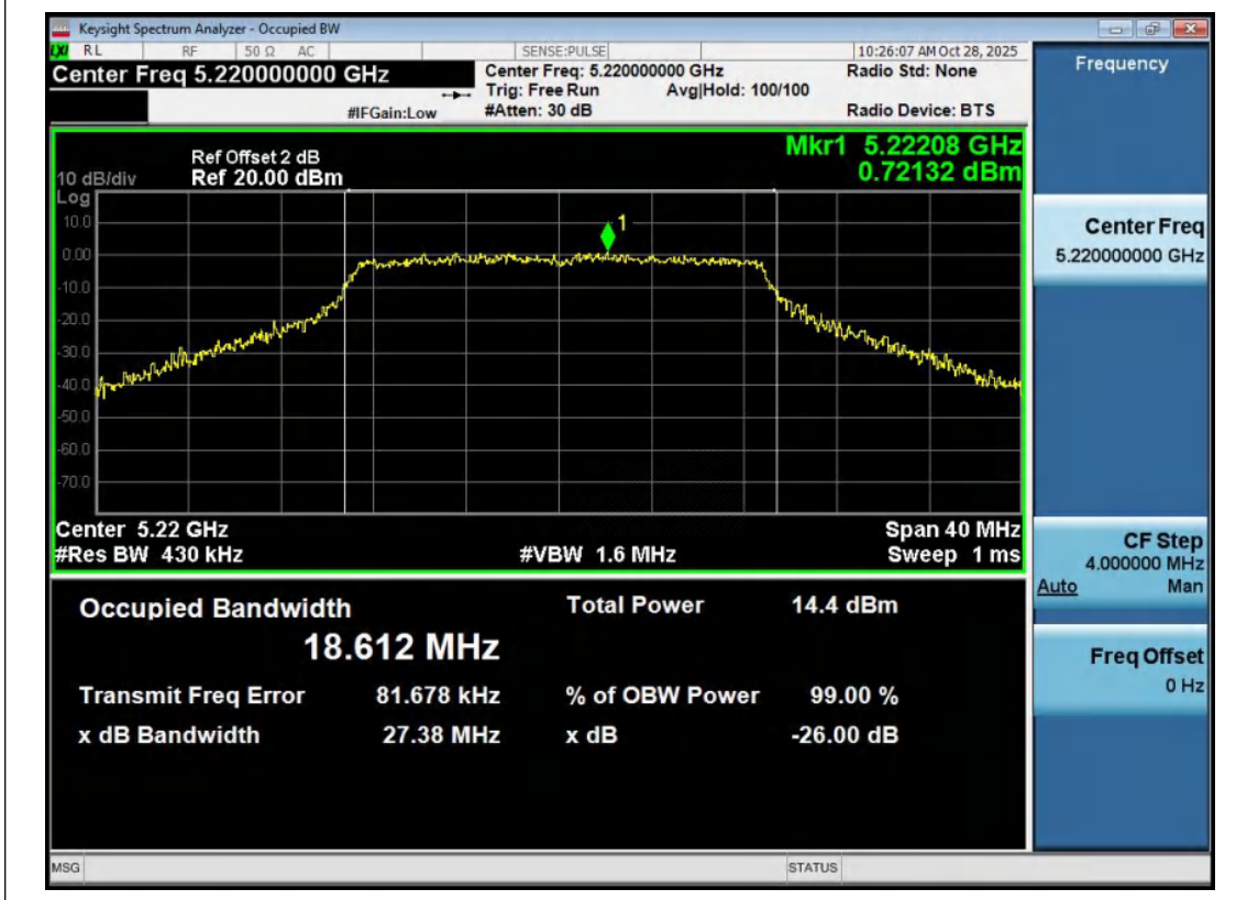
11N20MIMO-Ant2-5220
