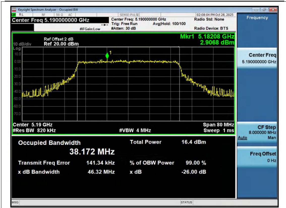
11AX40MIMO-Ant1-5190
