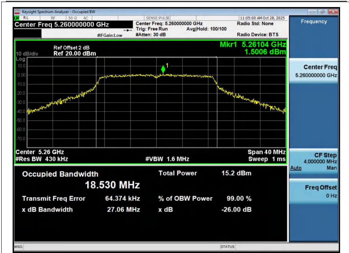
11AC20MIMO-Ant1-5260
