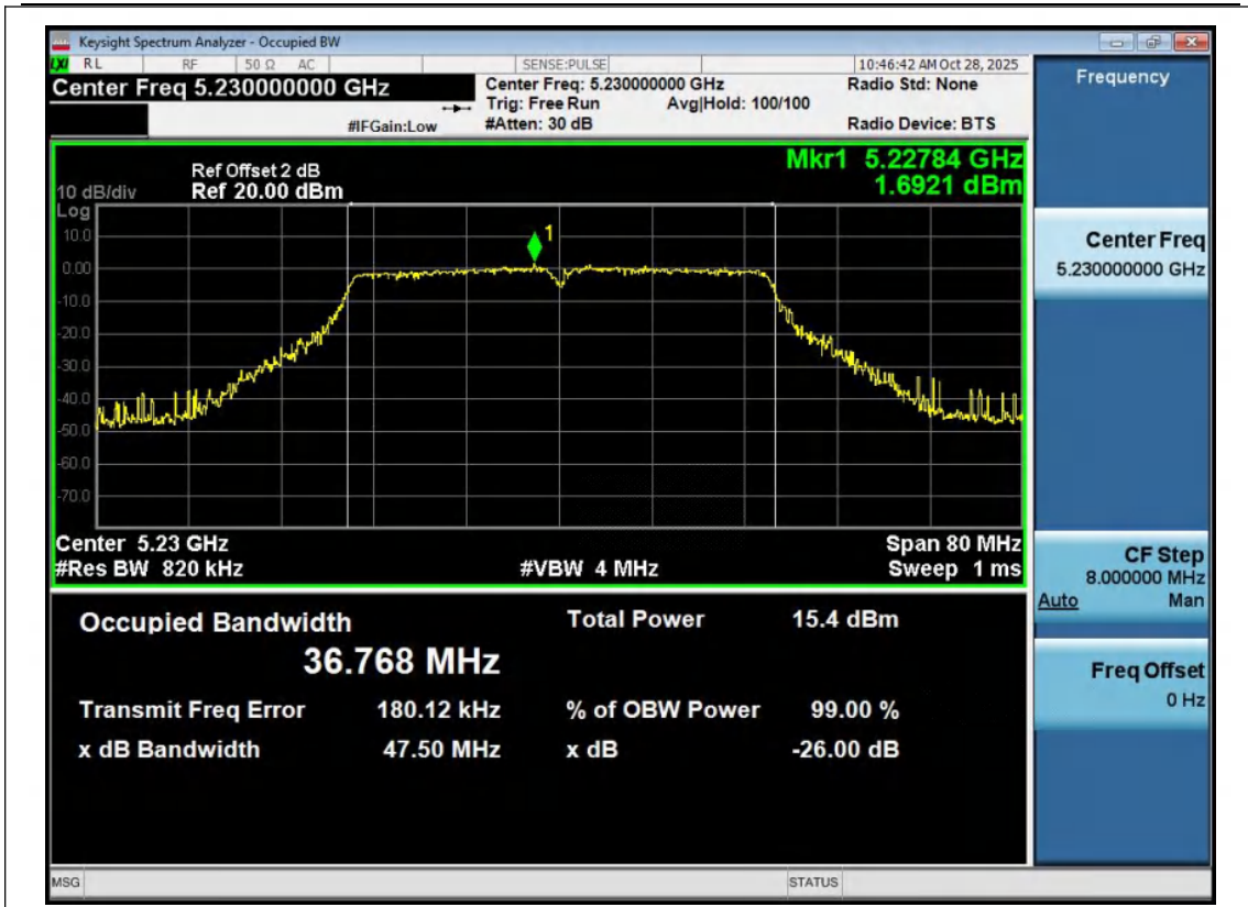
11N40MIMO-Ant1-5230
