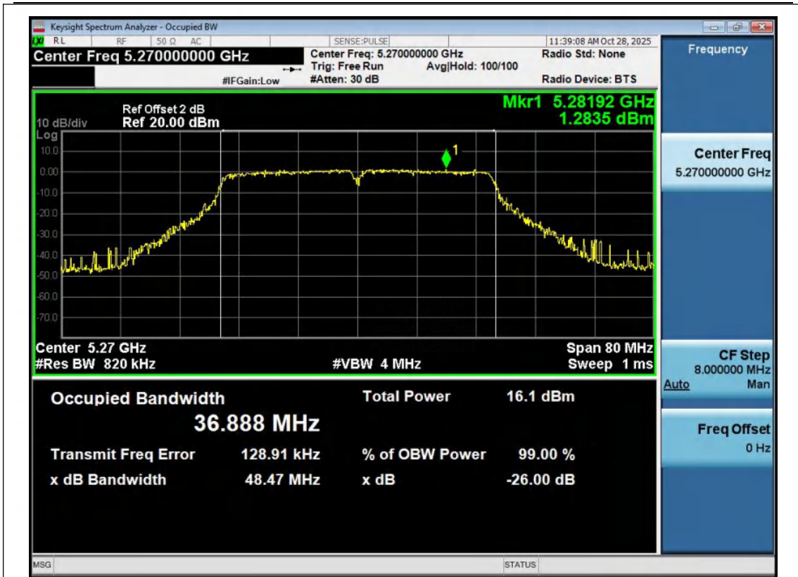
11AC40MIMO-Ant1-5270
