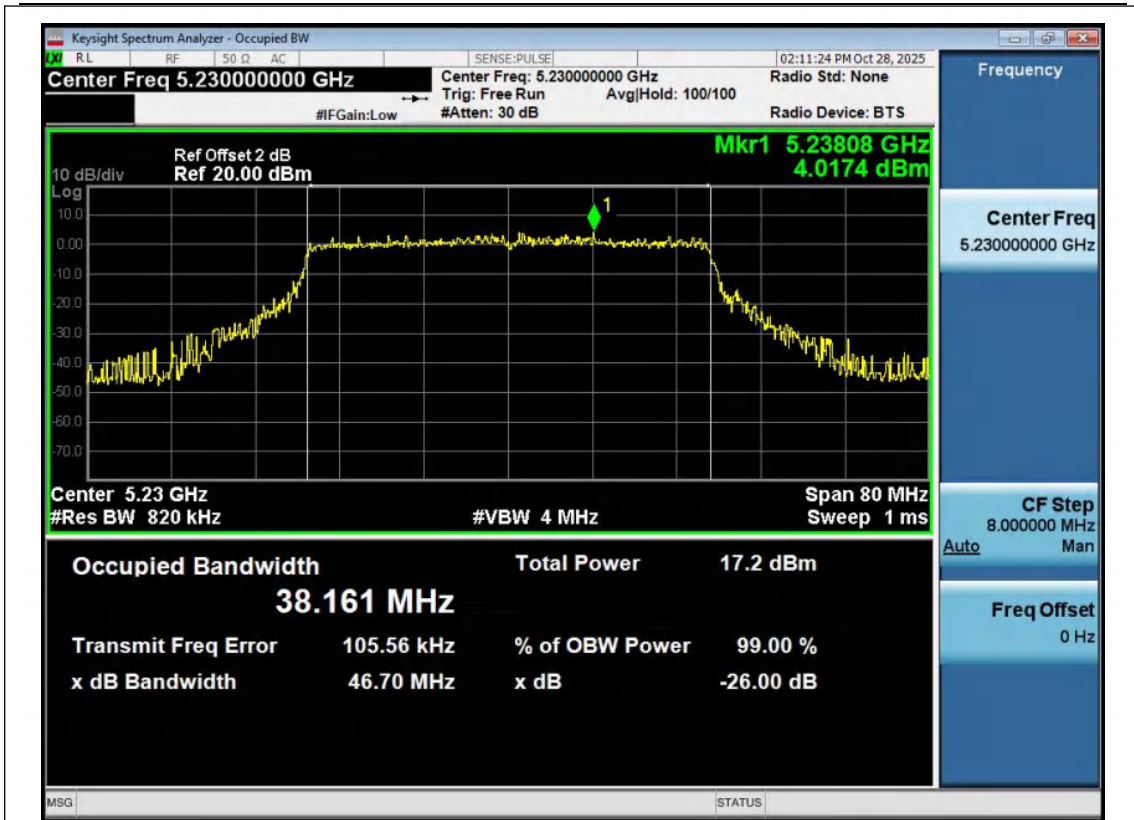
11AX40MIMO-Ant1-5230
