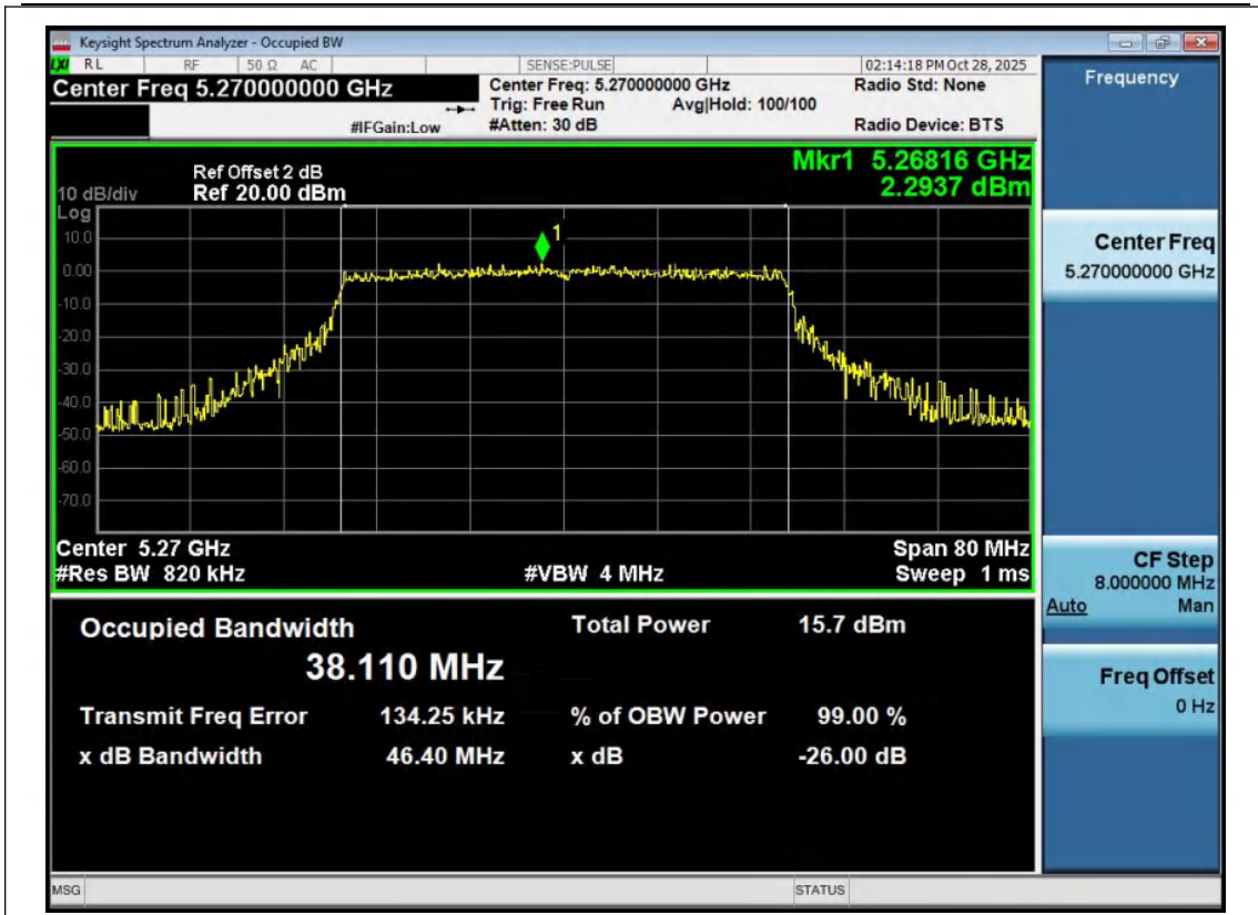
11AX40MIMO-Ant1-5270
