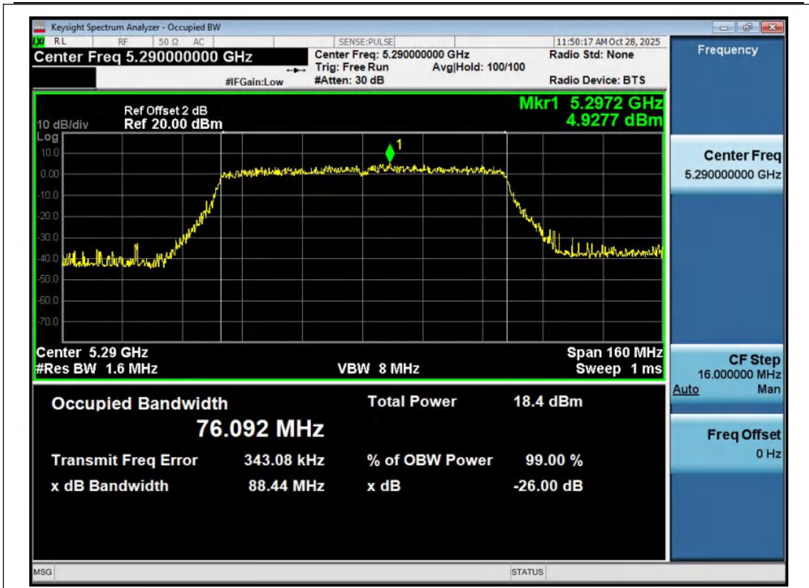
11AC80MIMO-Ant1-5290
