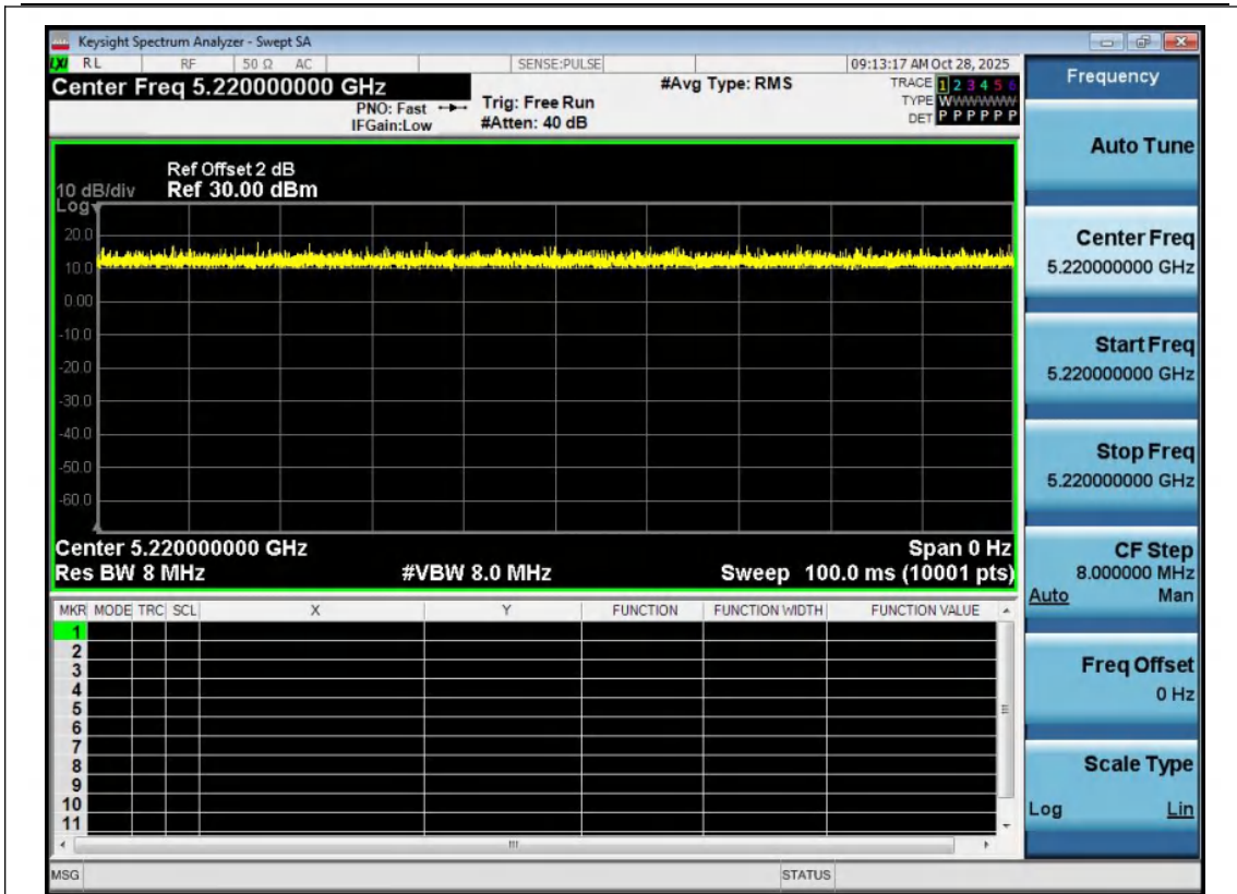
NTNV-11N20MIMO-Ant1-5220
