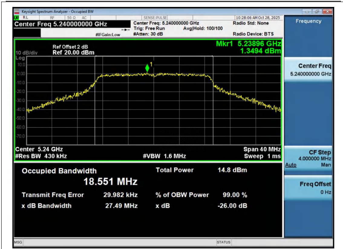
11N20MIMO-Ant1-5240
