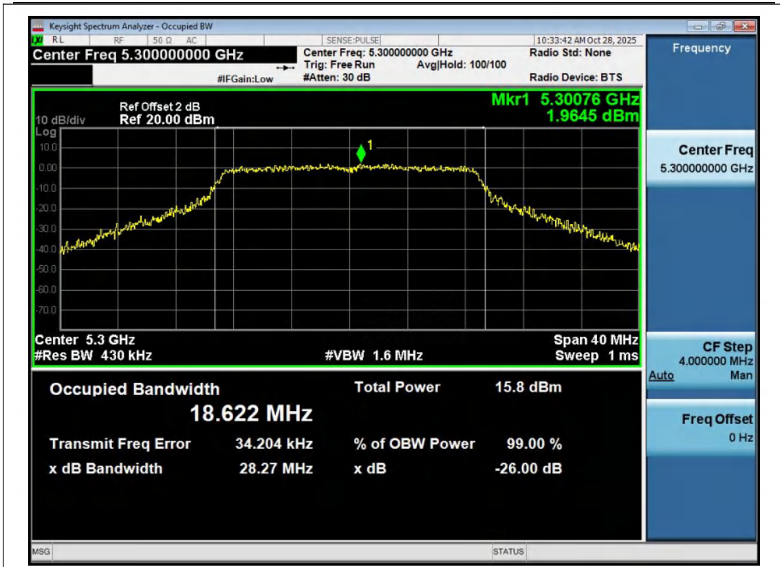
11N20MIMO-Ant1-5300
