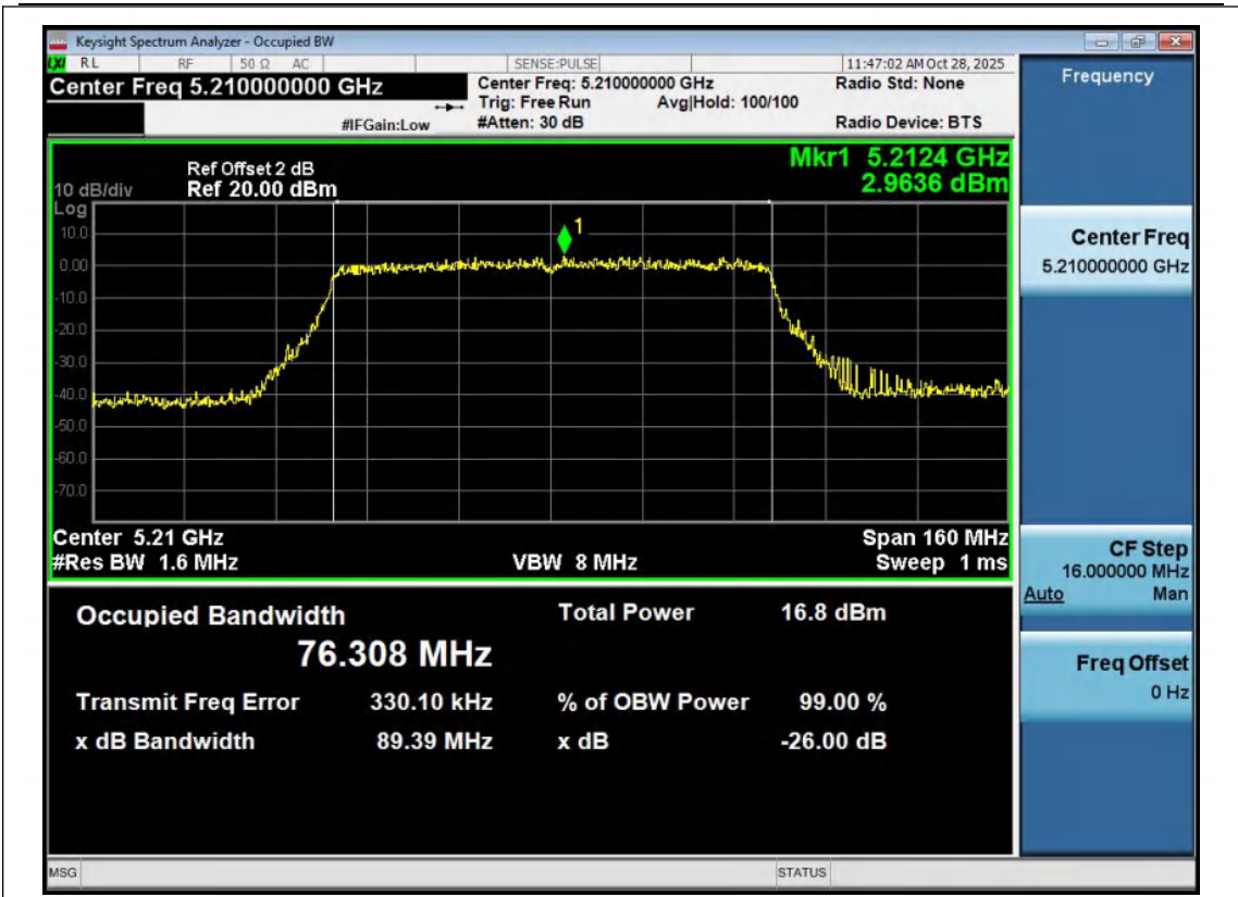
11AC80MIMO-Ant1-5210
