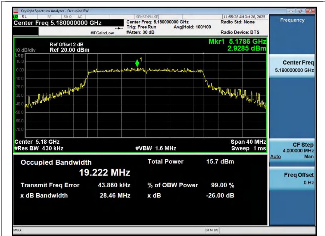
11AX20MIMO-Ant1-5180
