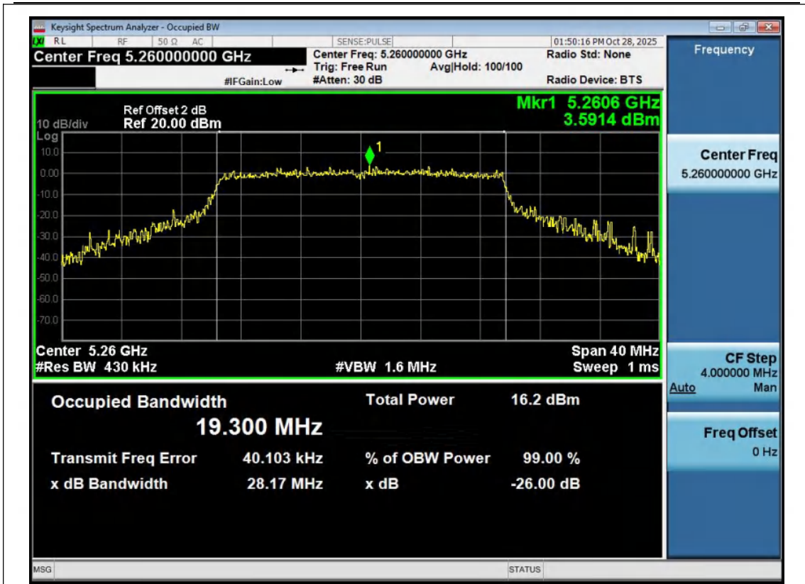
11AX20MIMO-Ant1-5260
