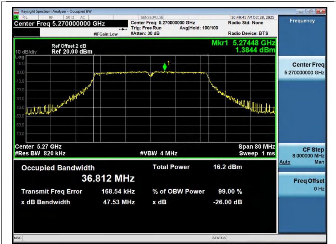
11N40MIMO-Ant1-5270
