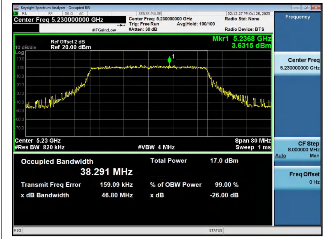
11AX40MIMO-Ant2-5230
