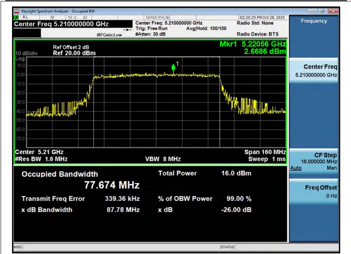
11AX80MIMO-Ant1-5210
