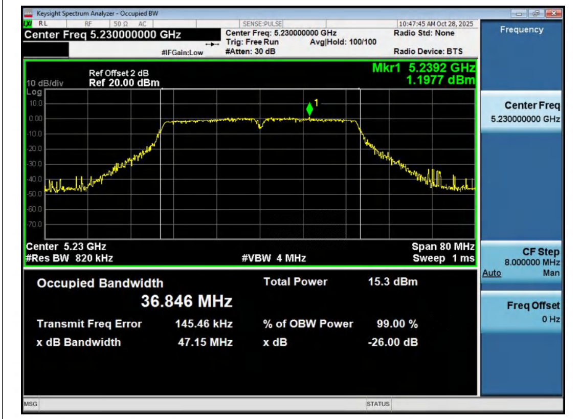
11N40MIMO-Ant2-5230
