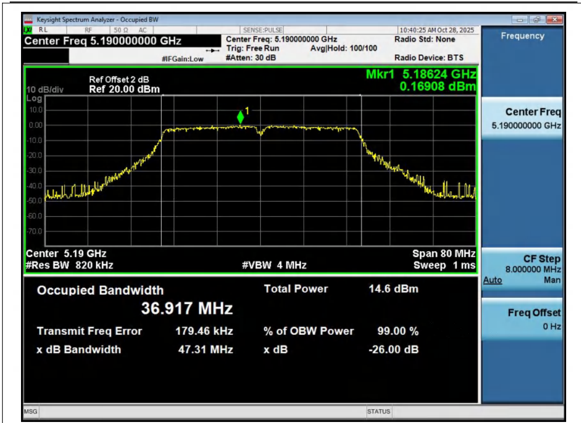
11N40MIMO-Ant1-5190
