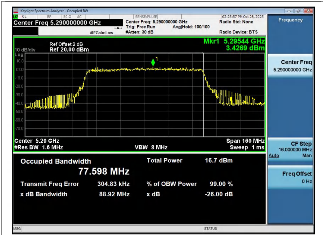
11AX80MIMO-Ant1-5290
