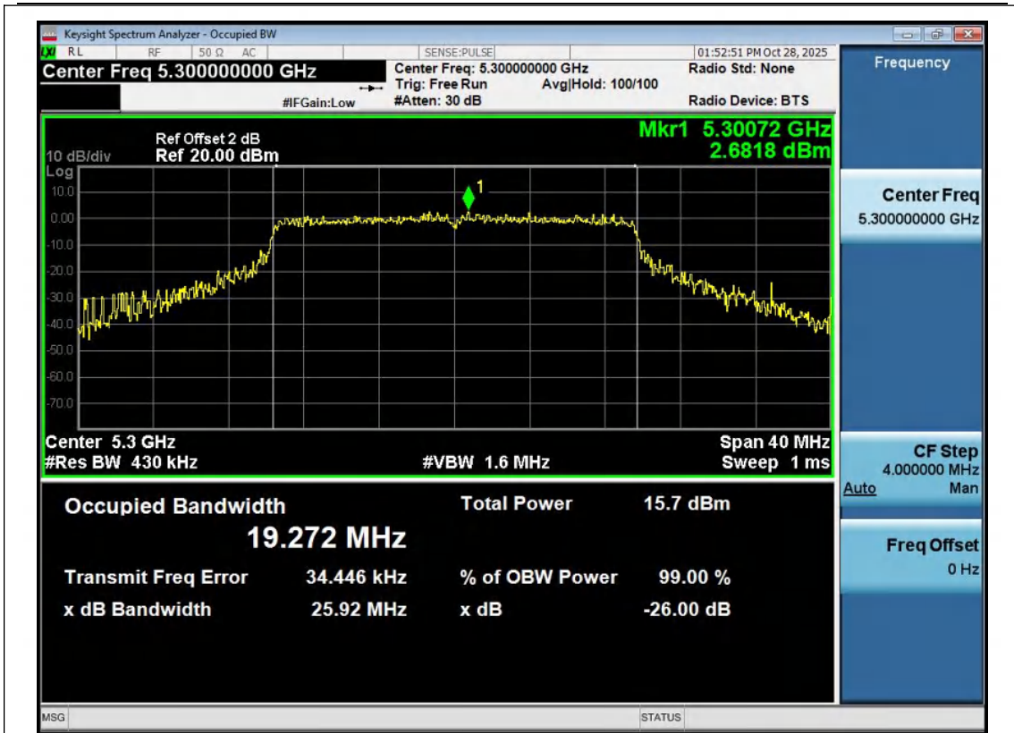
11AX20MIMO-Ant1-5300
