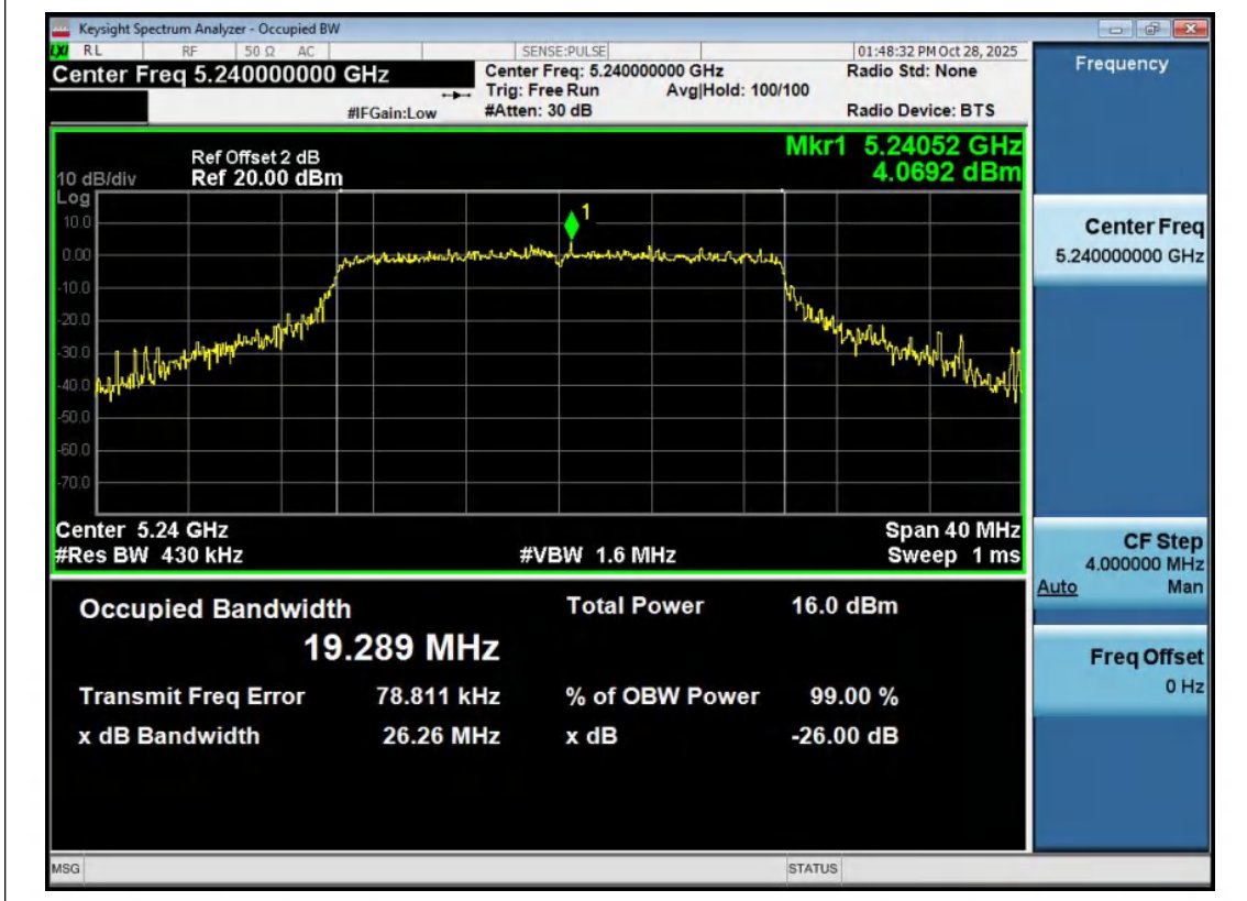
11AX20MIMO-Ant2-5240
