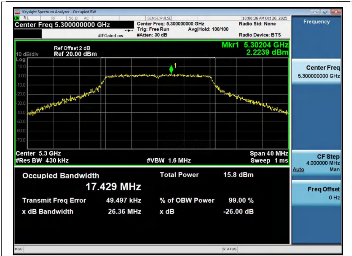
11A-Ant1-5300
