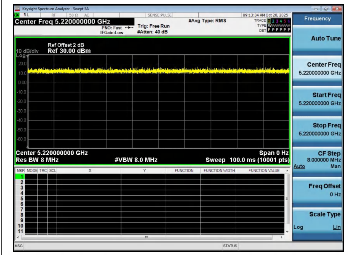
NTNV-11N20MIMO-Ant2-5220
