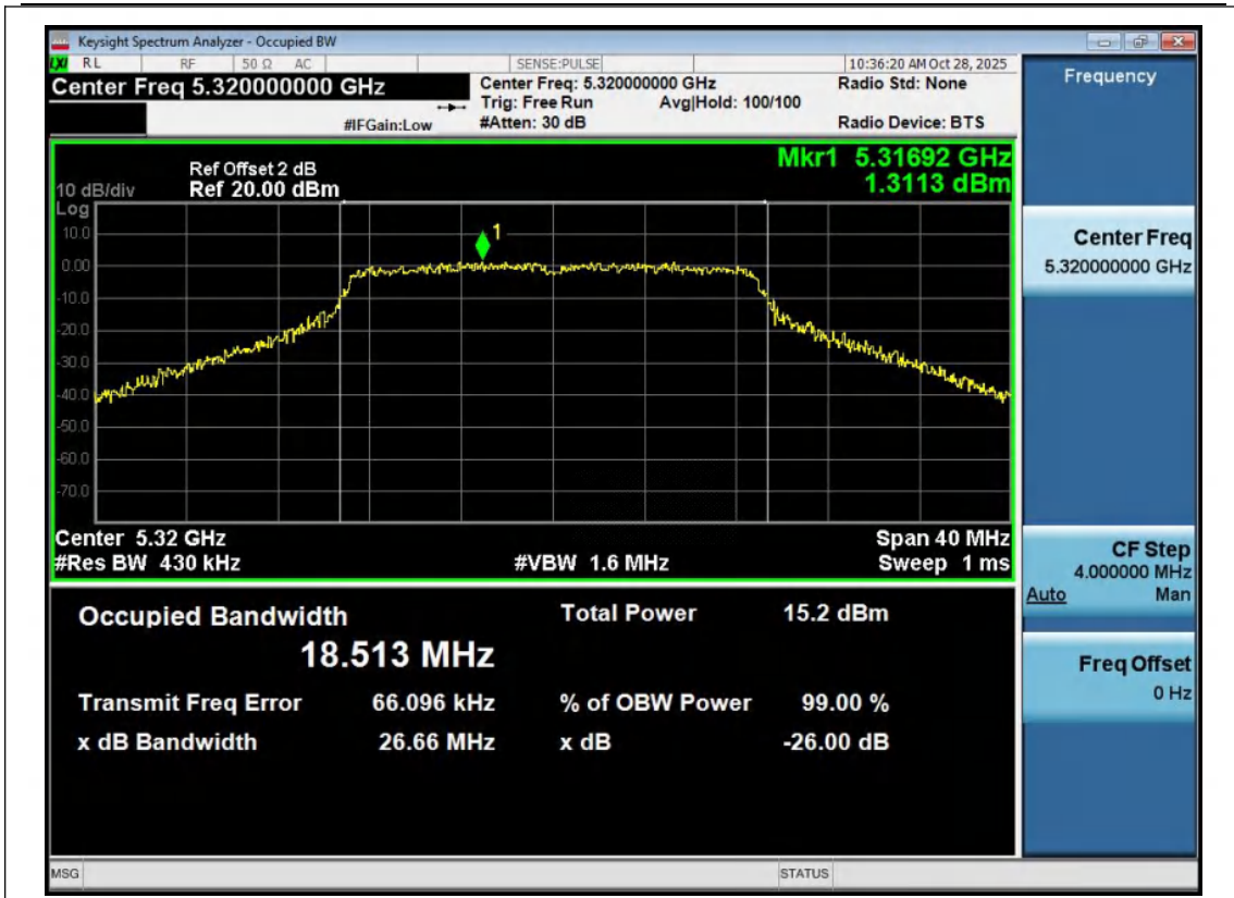
11N20MIMO-Ant1-5320
