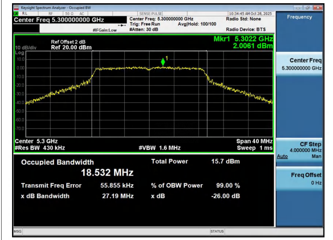
11N20MIMO-Ant2-5300
