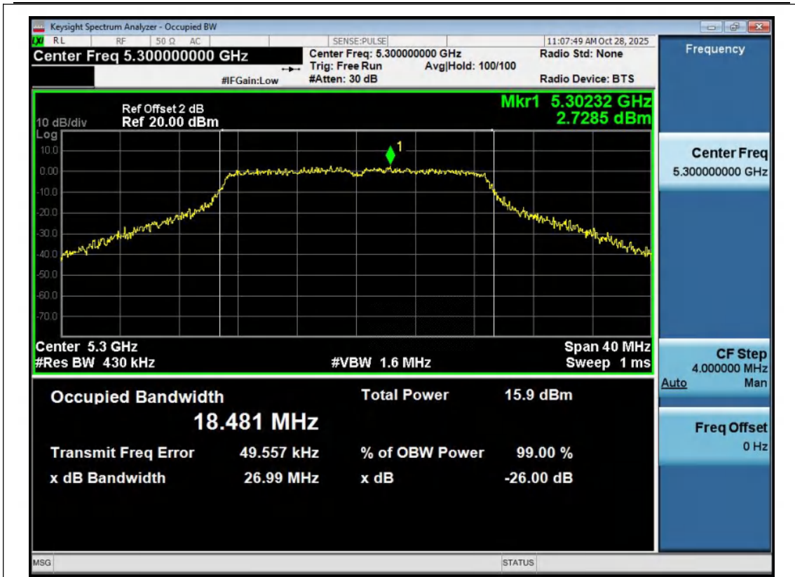
11AC20MIMO-Ant1-5300
