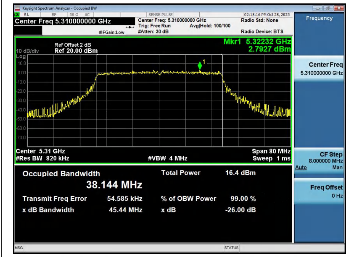
11AX40MIMO-Ant2-5310
