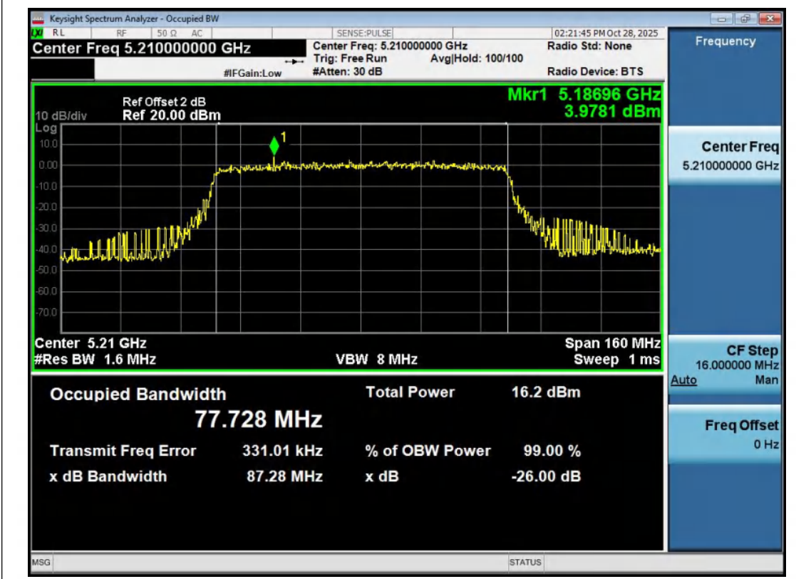
11AX80MIMO-Ant2-5210
