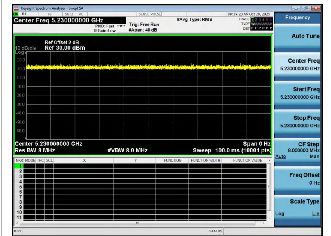
NTNV-11AX40MIMO-Ant2-5230
