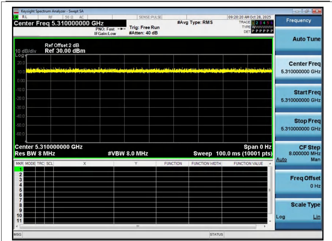
NTNV-11N40MIMO-Ant1-5310
