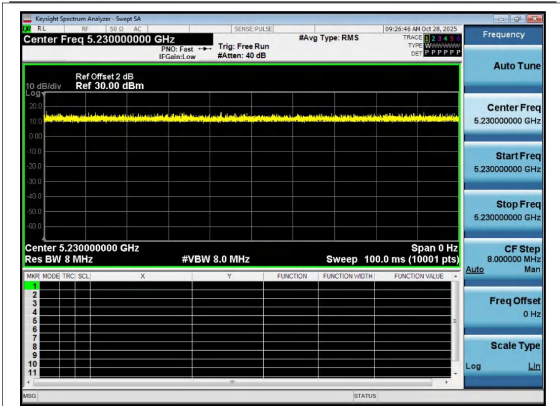
NTNV-11AC40MIMO-Ant1-5230
