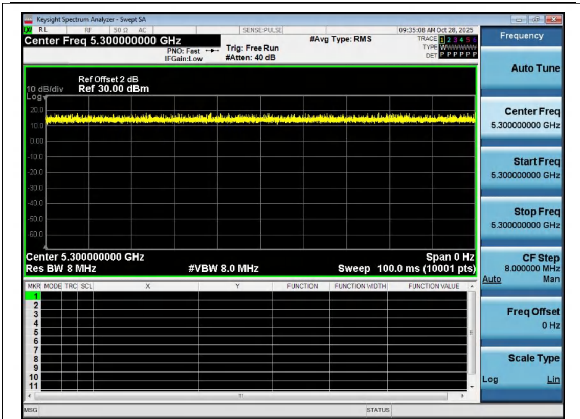
NTNV-11AX20MIMO-Ant1-5300
