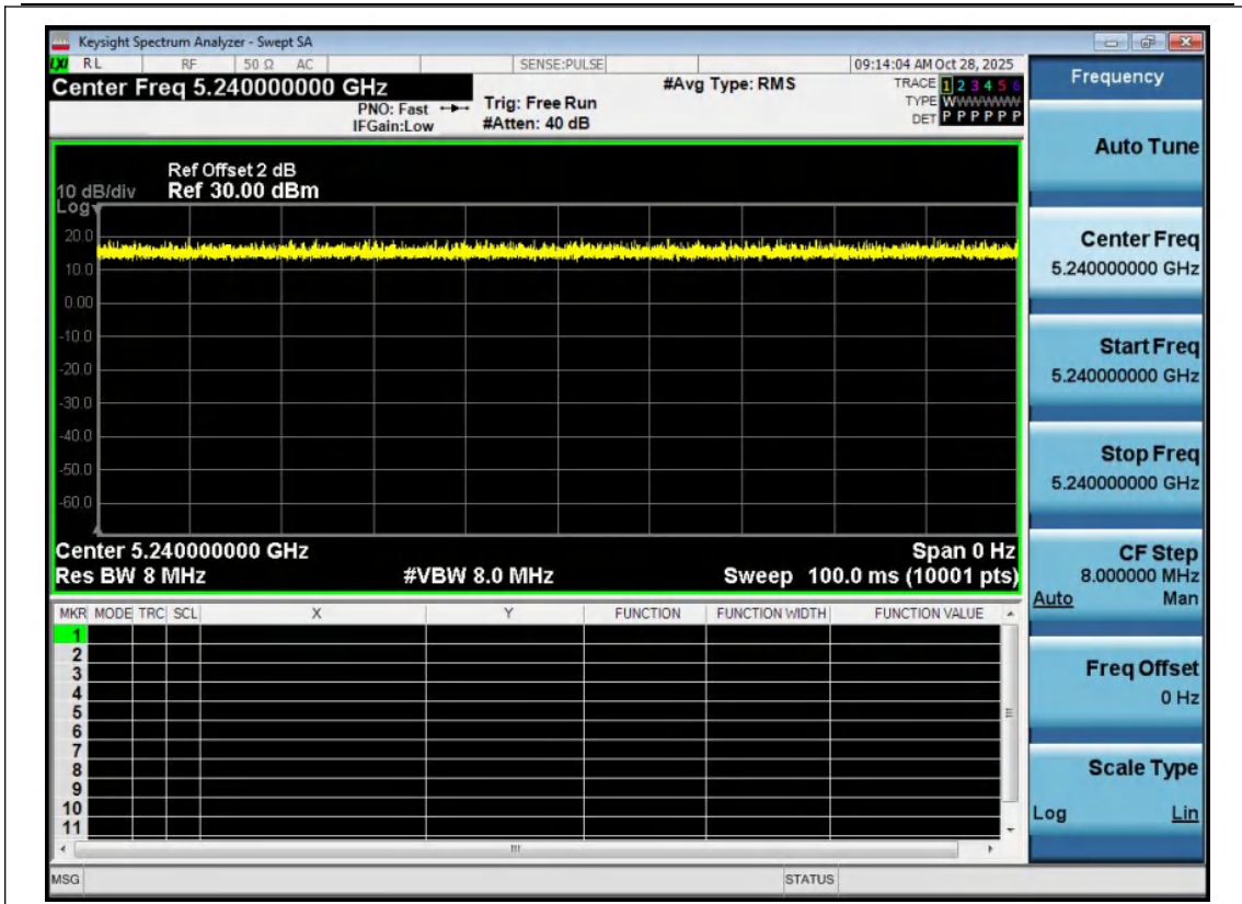
NTNV-11N20MIMO-Ant1-5240
