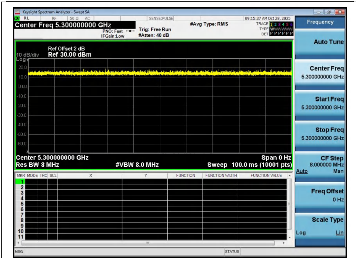
NTNV-11N20MIMO-Ant1-5300
