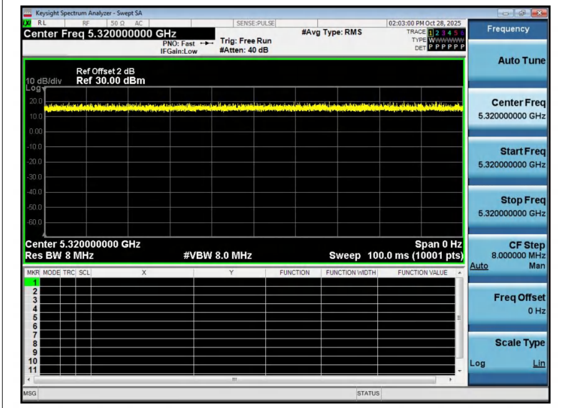
NTNV-11AX20MIMO-Ant1-5320
