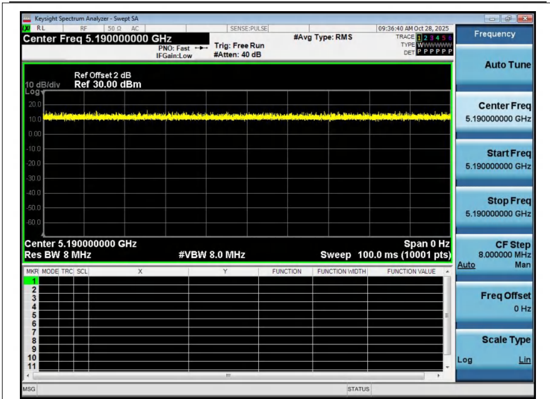
NTNV-11AX40MIMO-Ant1-5190
