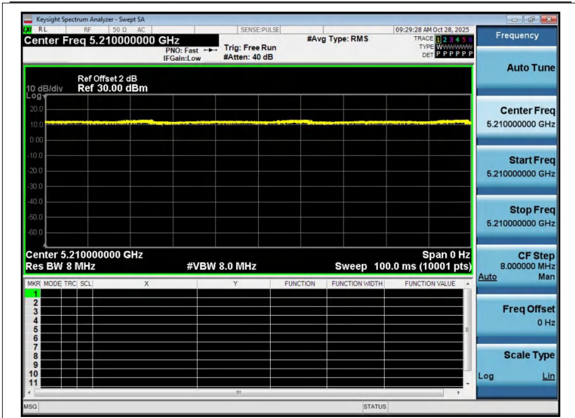
NTNV-11AC80MIMO-Ant1-5210
