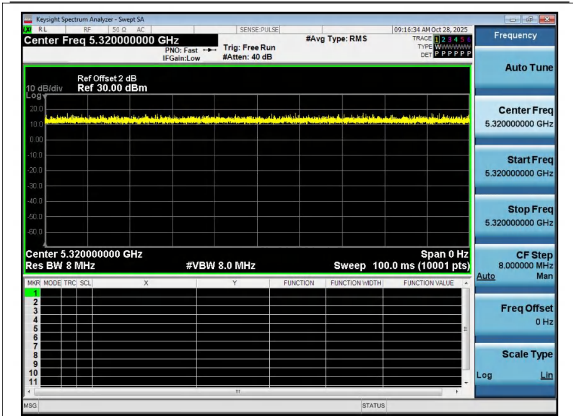
NTNV-11N20MIMO-Ant1-5320
