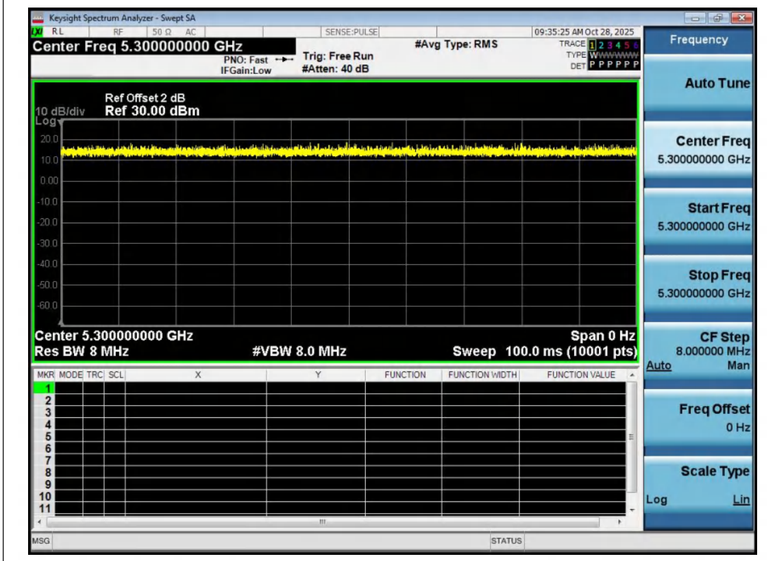
NTNV-11AX20MIMO-Ant2-5300
