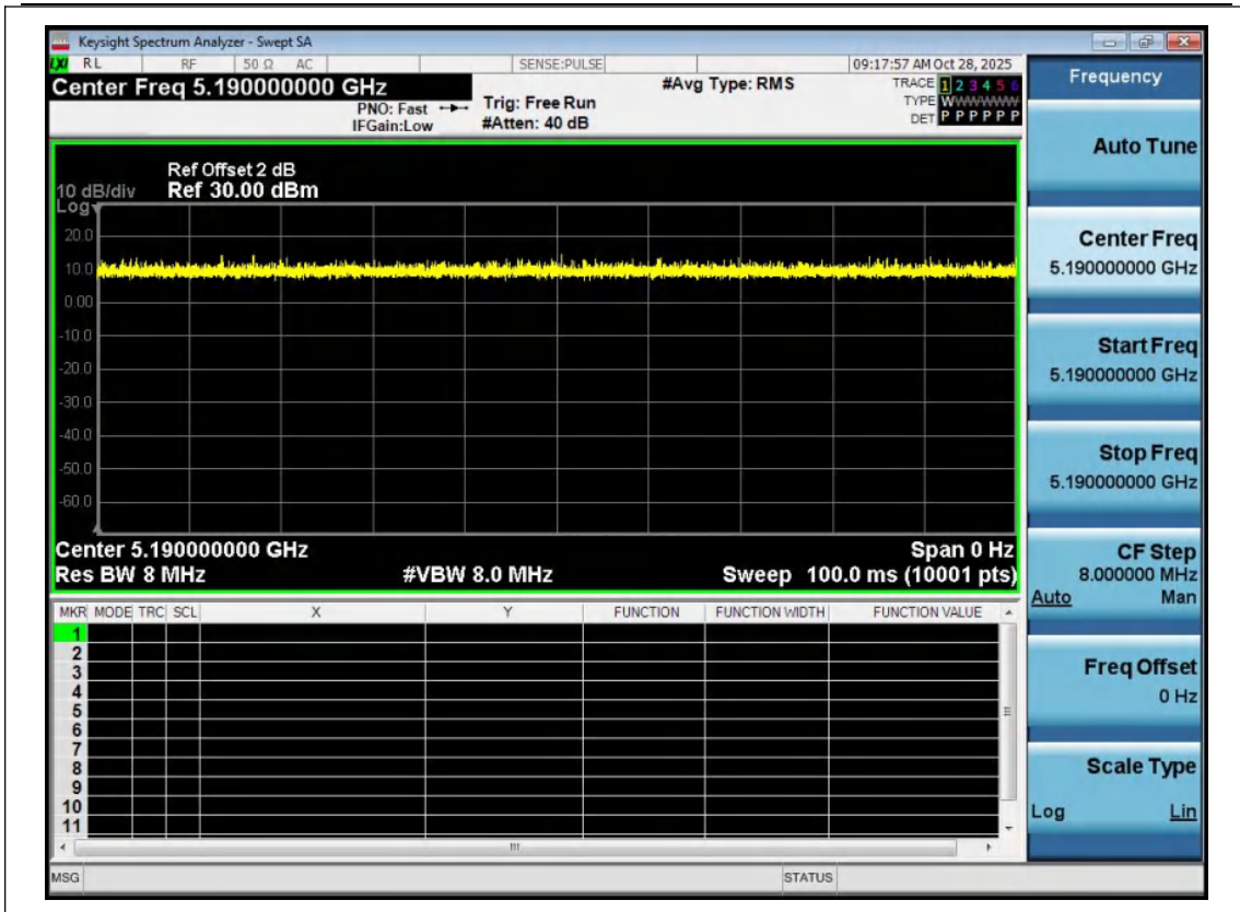
NTNV-11N40MIMO-Ant1-5190
