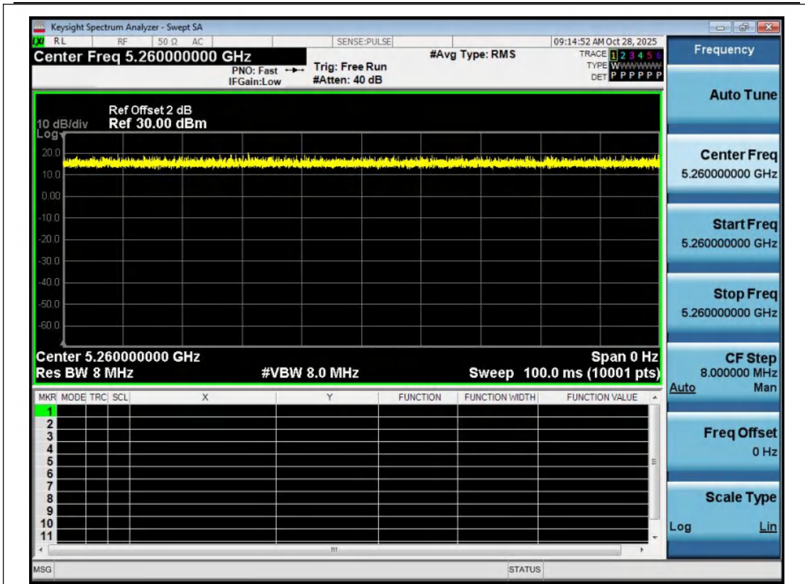
NTNV-11N20MIMO-Ant1-5260
