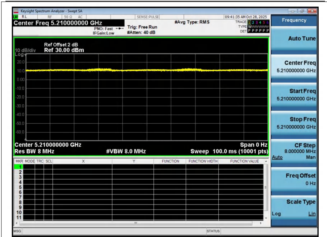
NTNV-11AX80MIMO-Ant1-5210
