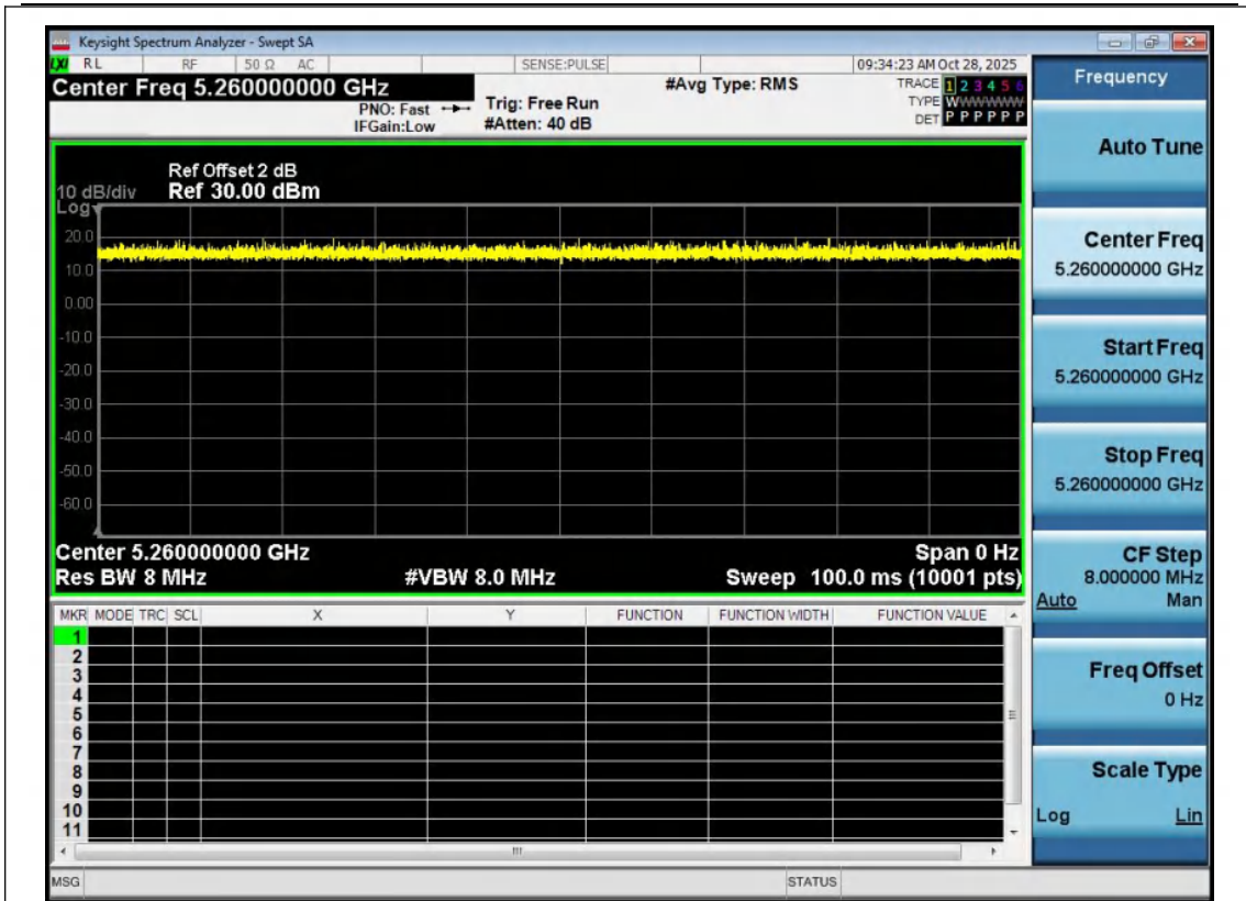
NTNV-11AX20MIMO-Ant1-5260
