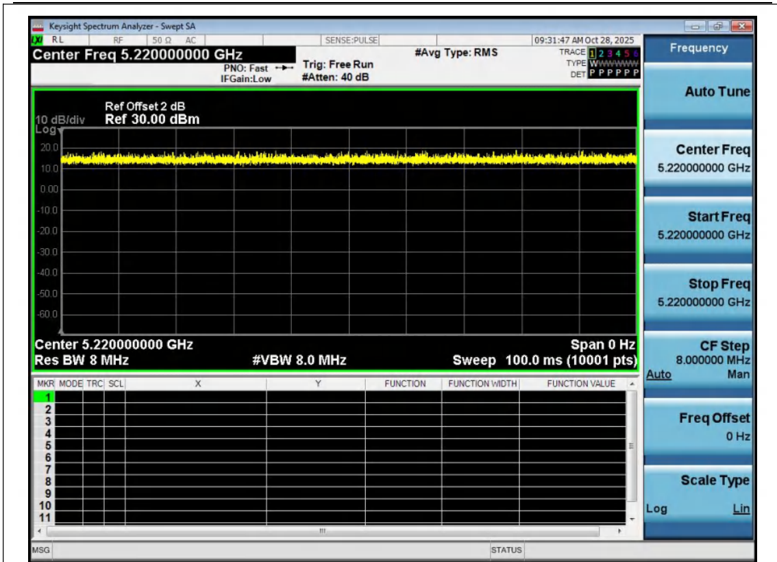
NTNV-11AX20MIMO-Ant1-5220
