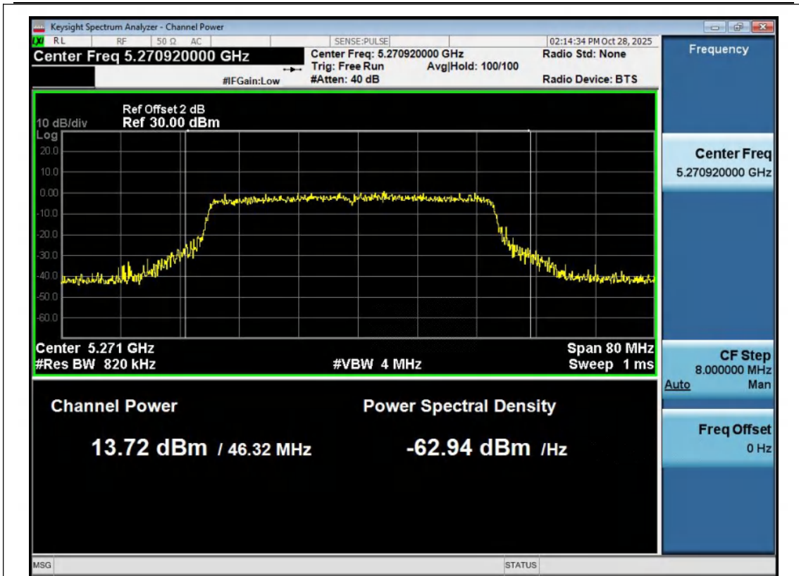
11AX40MIMO-Ant1-5270-PASS
