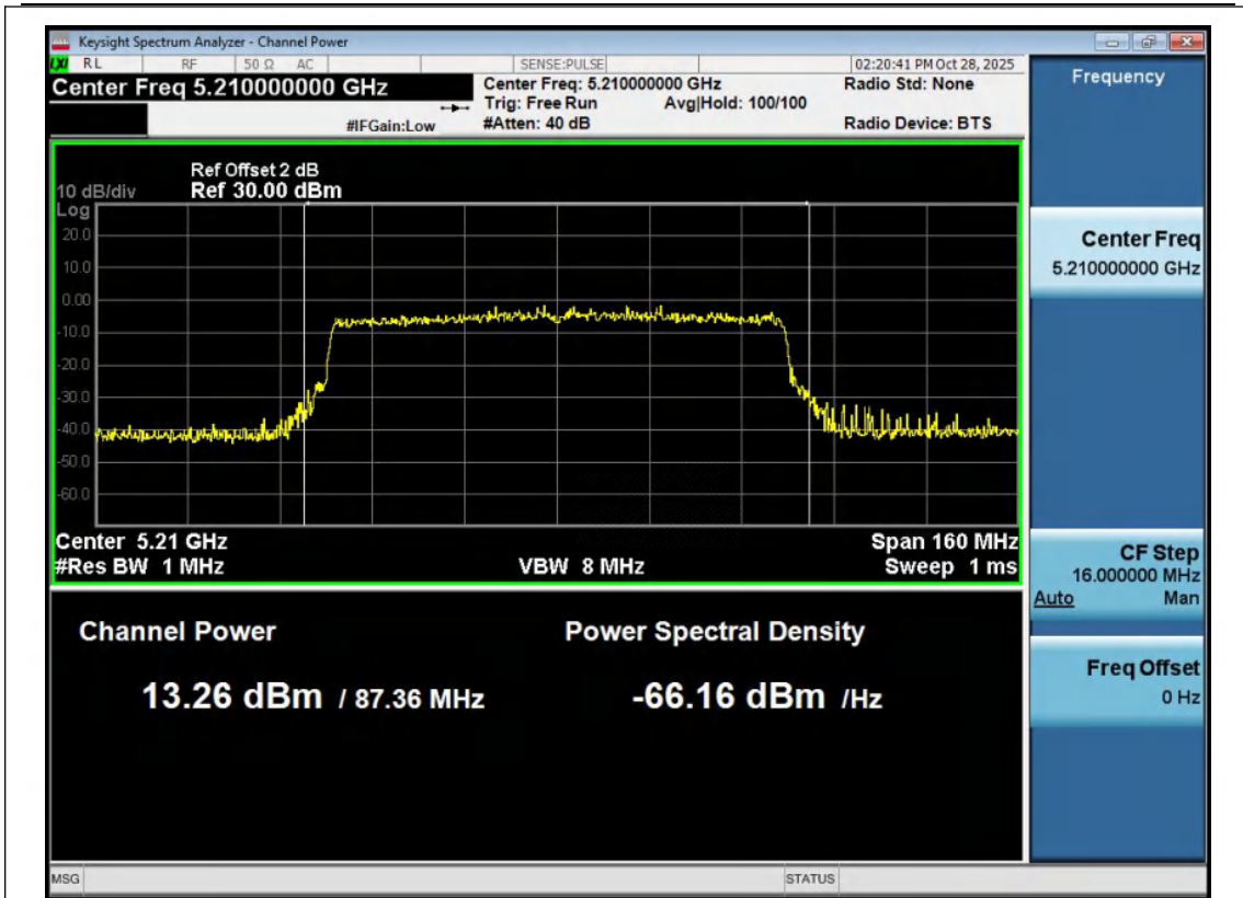
11AX80MIMO-Ant1-5210-PASS
