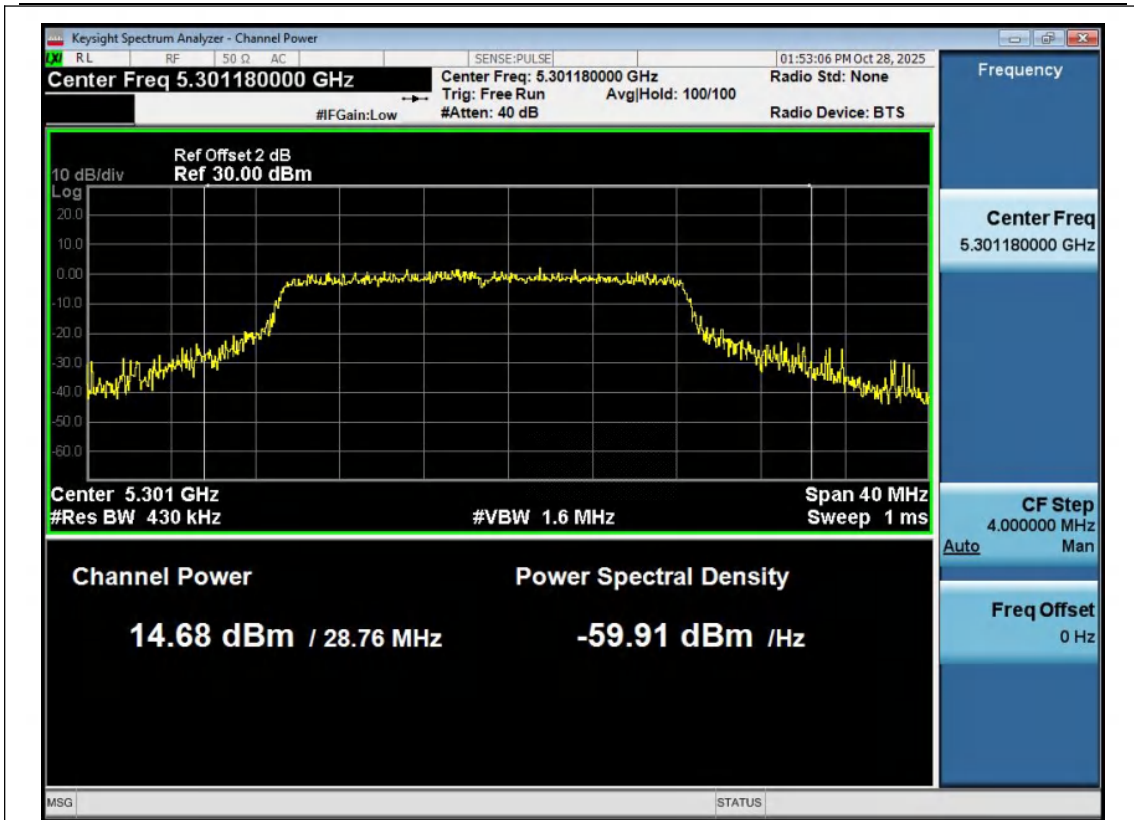
11AX20MIMO-Ant1-5300-PASS
