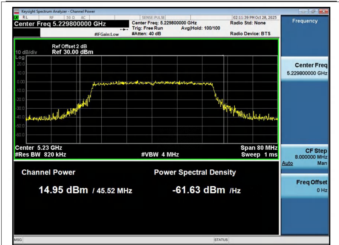
11AX40MIMO-Ant1-5230-PASS
