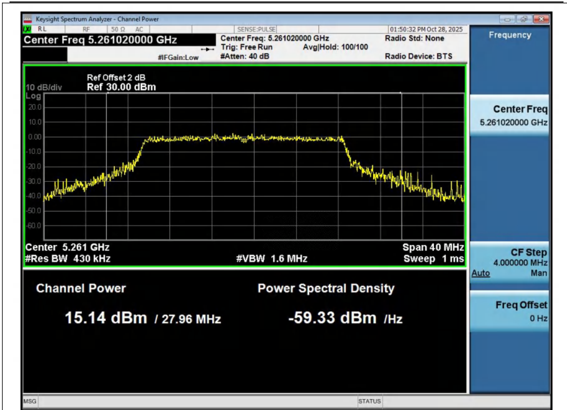
11AX20MIMO-Ant1-5260-PASS
