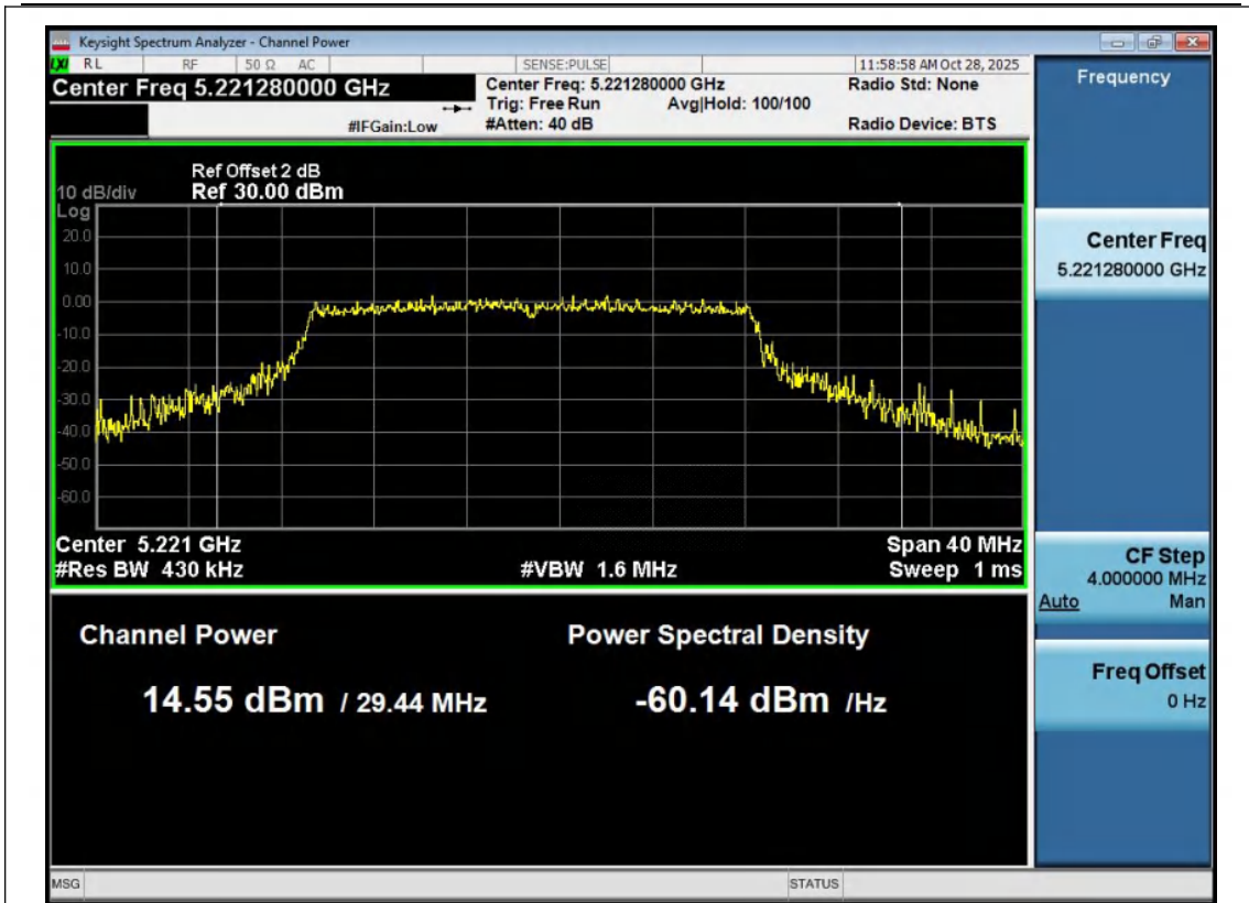
11AX20MIMO-Ant1-5220-PASS
