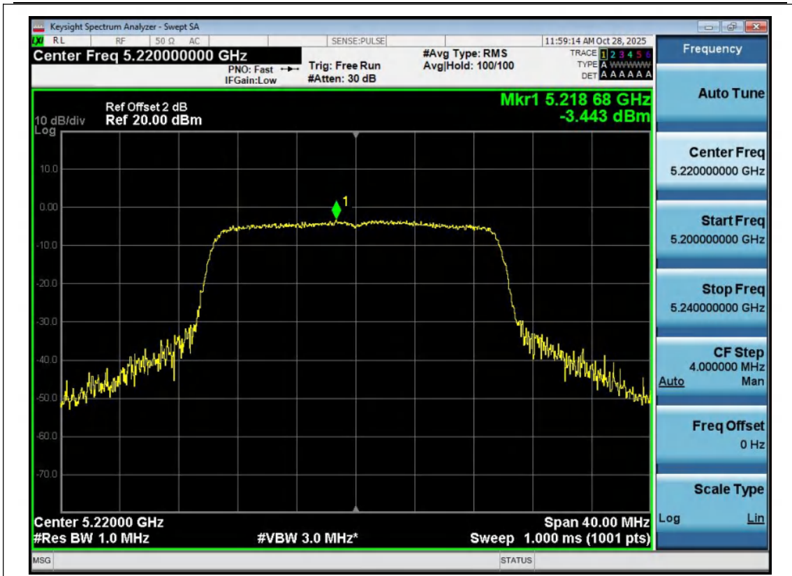
11AX20MIMO-Ant1-5220-PASS
