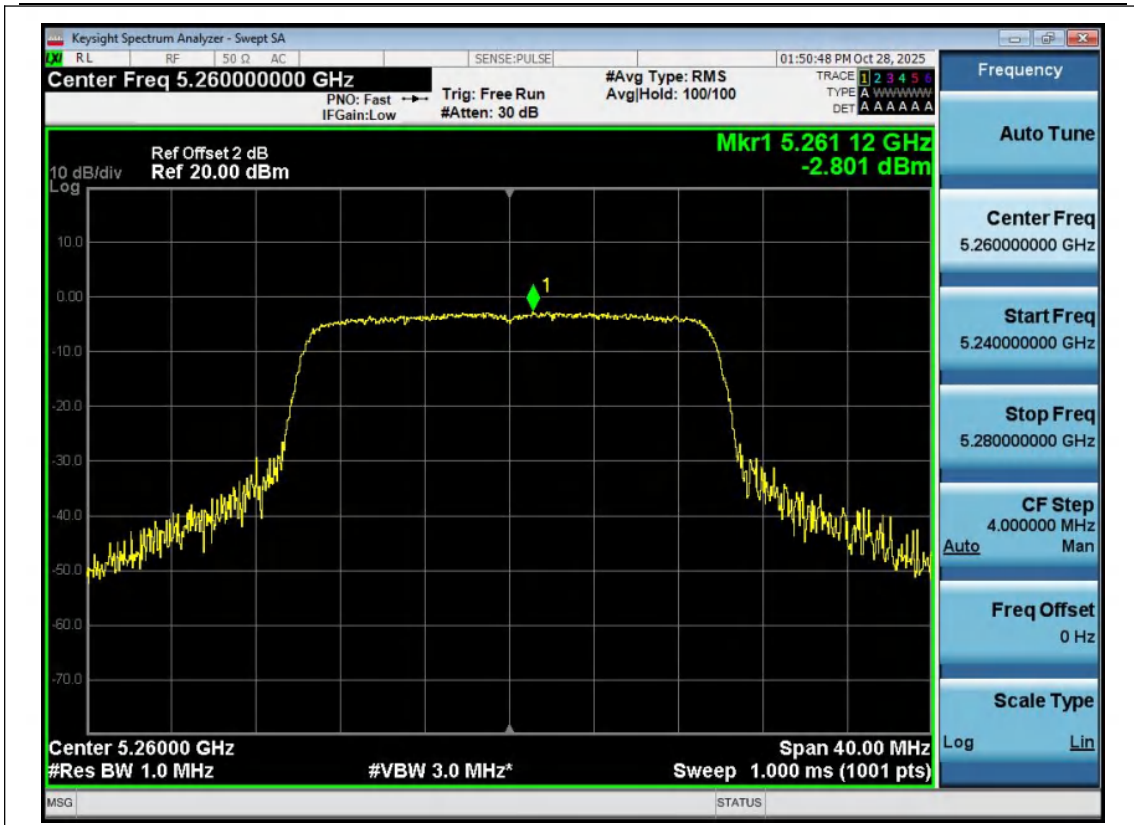
11AX20MIMO-Ant1-5260-PASS
