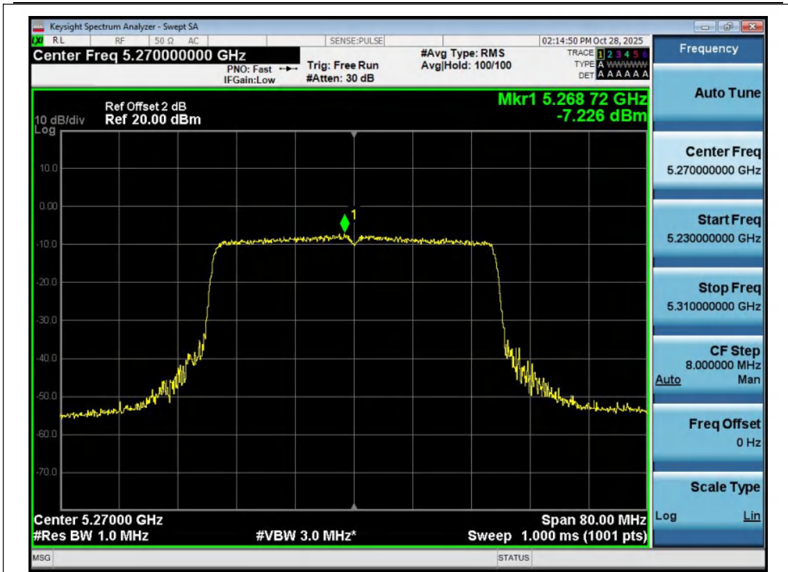
11AX40MIMO-Ant1-5270-PASS
