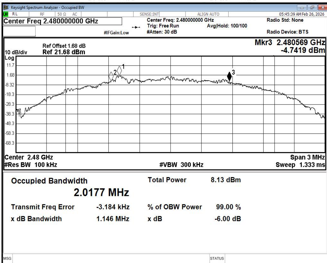
-6dB Bandwidth NVNT BLE 2M 2480MHz Ant1
