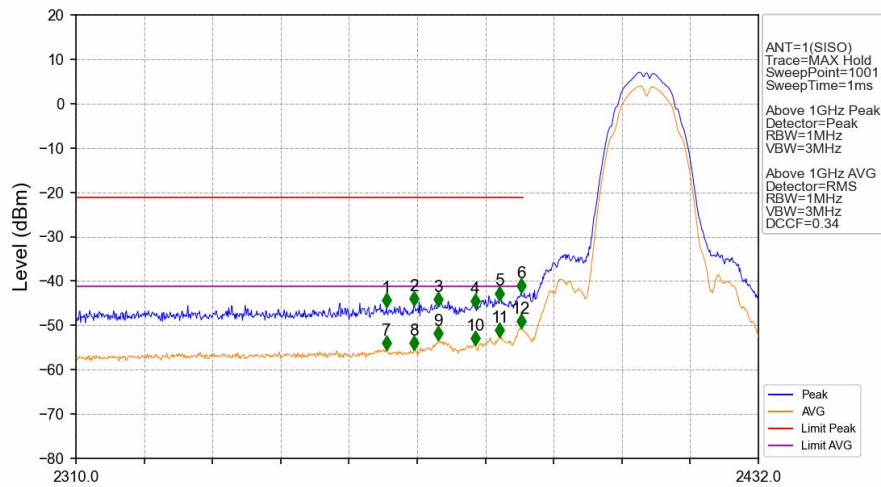
802.11b_LCH_2412MHz_Ant1 (SISO)_NTNV
