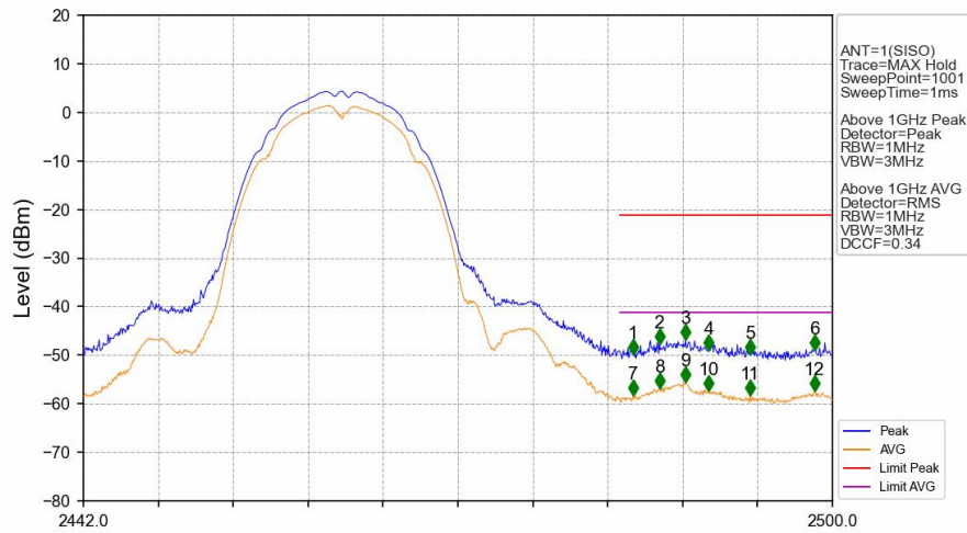
802.11b_HCH_2462MHz_Ant1 (SISO)_NTNV
