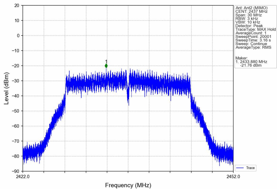
802.11n(HT20)_MCH_2437MHz_MIMO_NTNV
