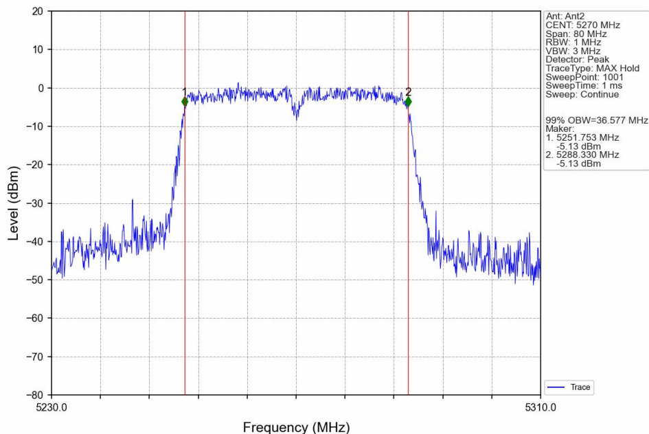
802.11ac(VHT40)_LCH_5270MHz_Ant2_NTNV
