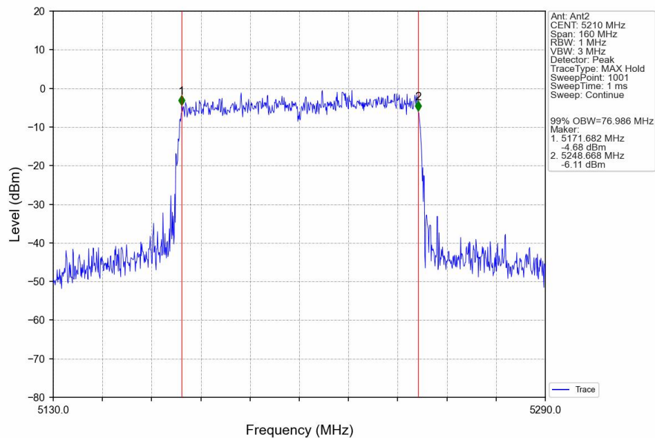
802.11ax(HEW80)_MCH_5210MHz_SU_ / _Ant2_NTNV
