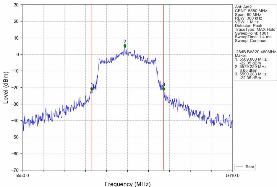
802.11a_MCH_5580MHz_Ant2_NTNV
