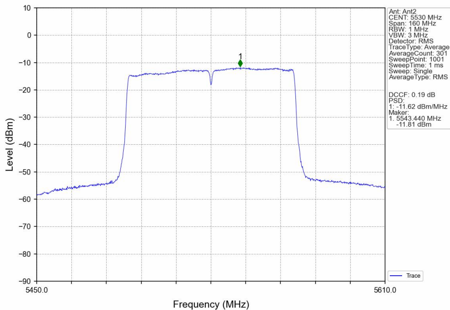
802.11ac(VHT80)_LCH_5530MHz_Ant2_NTNV
