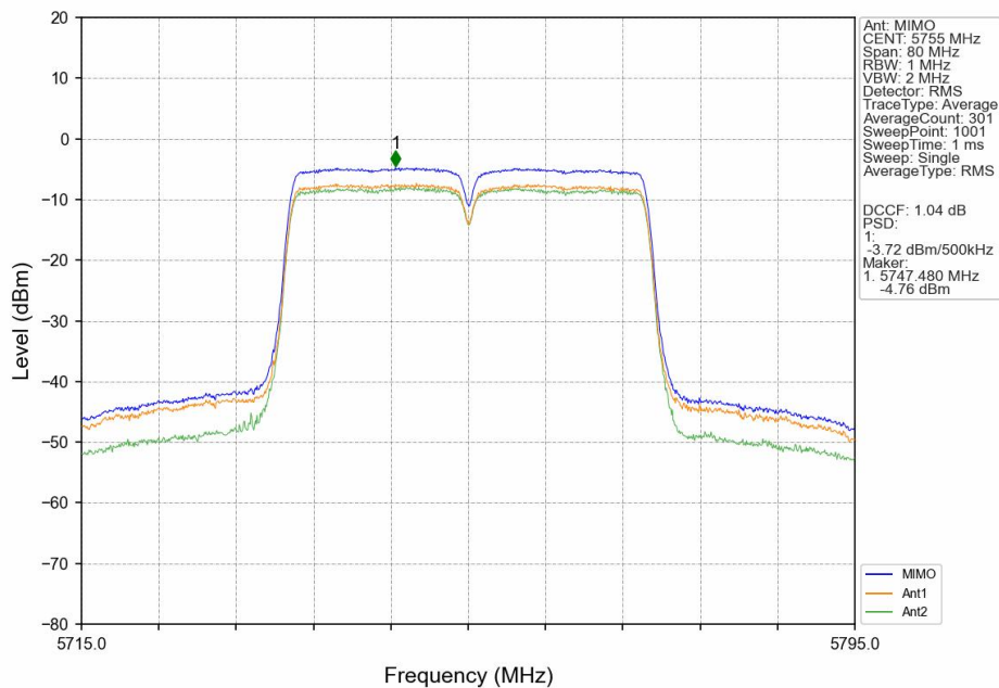
802.11n(HT40)_LCH_5755MHz_MIMO_NTNV
