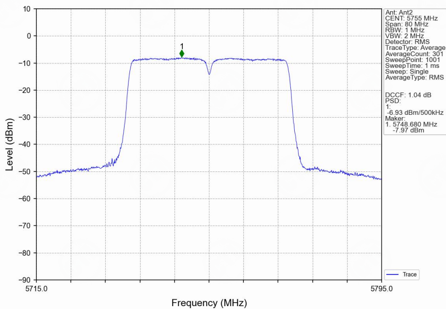
802.11n(HT40)_LCH_5755MHz_MIMO_NTNV
