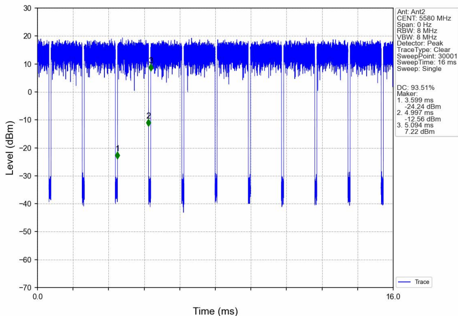
802.11a_MCH_5580MHz_Ant2_NTNV
