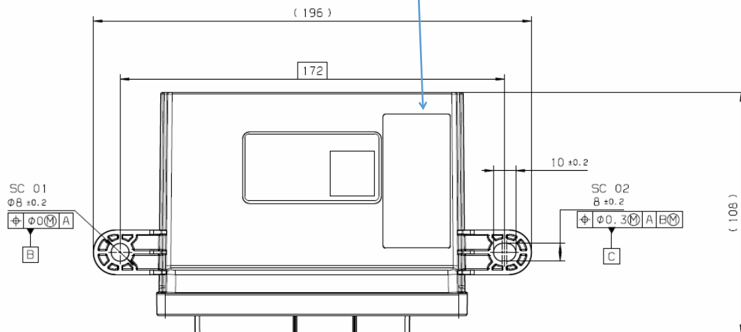
FRONT VIEW SCALE: 1:1
