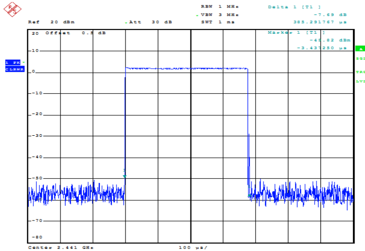
GFSK_Hopping_DH1 0.385ms
