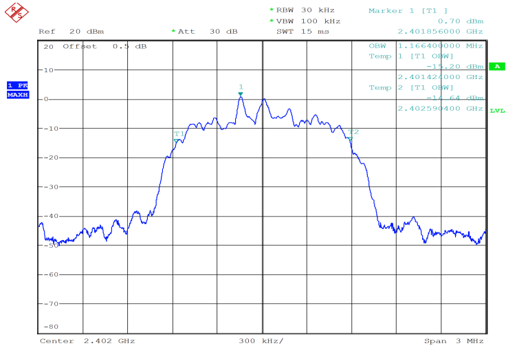
\pi/4 -DQPSK_Low 1.166 MHz
