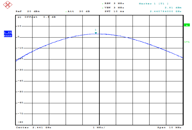
\pi/4 -DQPSK_Middle 2.81 dBm
