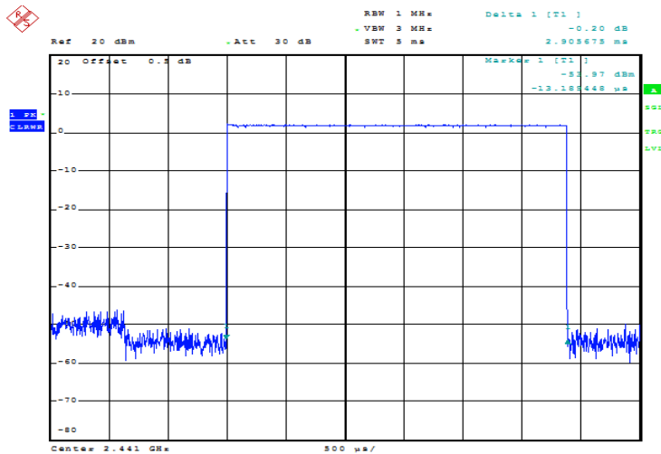
GFSK_Hopping_DH5 2.906ms
