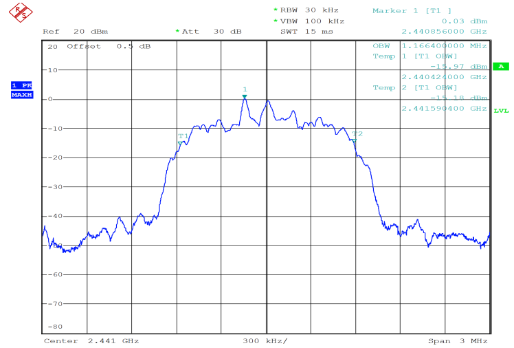
\pi/4 -DQPSK_Middle 1.166 MHz
