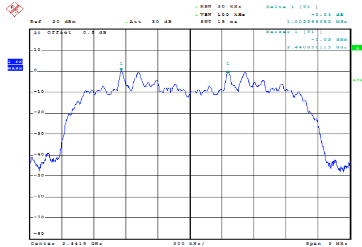
\pi/4 -DQPSK_Middle 1.002 MHz
