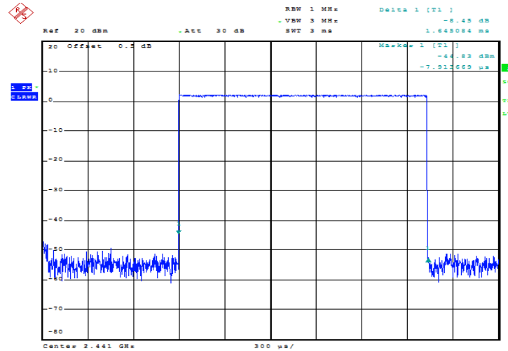
GFSK_Hopping_DH3 1.645ms
