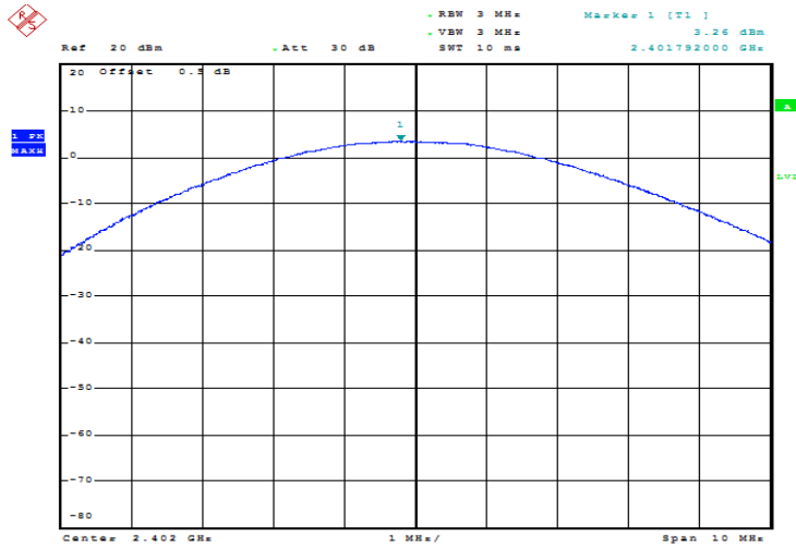
\pi/4 -DQPSK_Low 3.26 dBm
