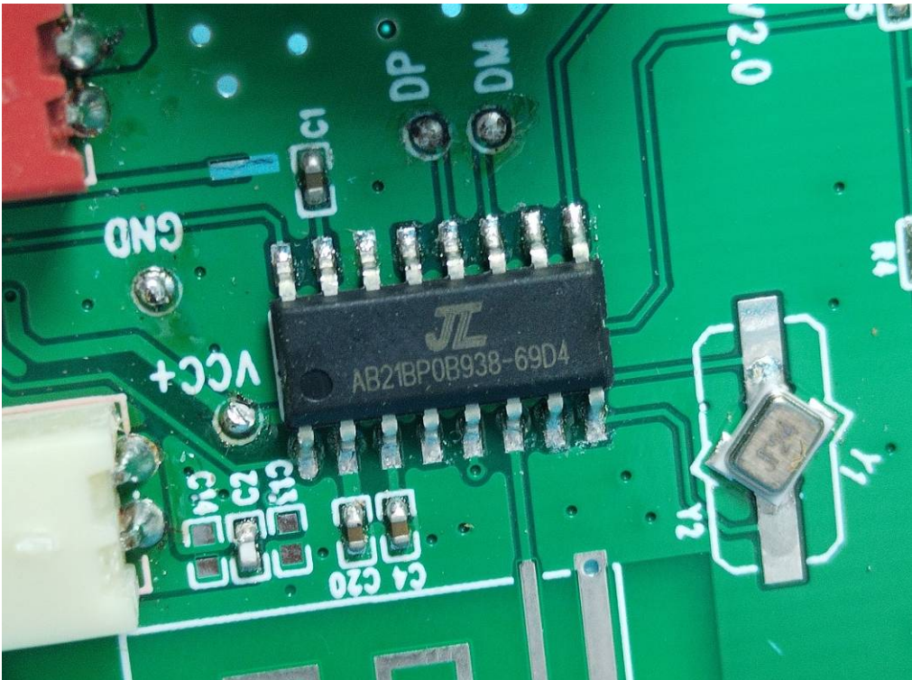
BT ANT
