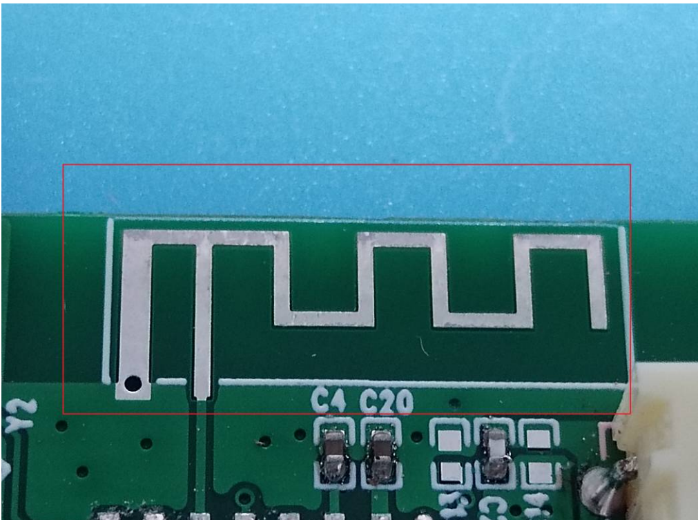
BT ANT
