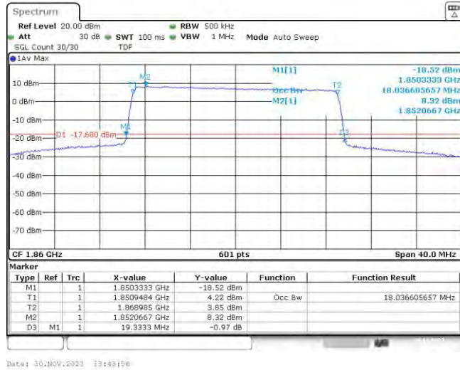
Band25-20MHz-QPSK-26365-100RB#0
