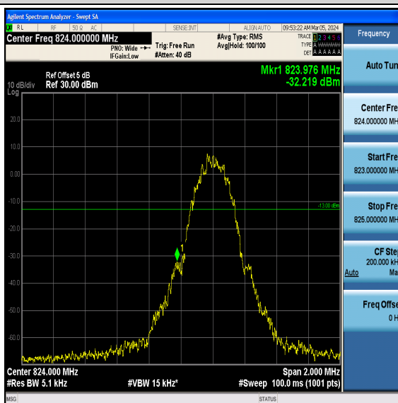
EGPRS850-128
