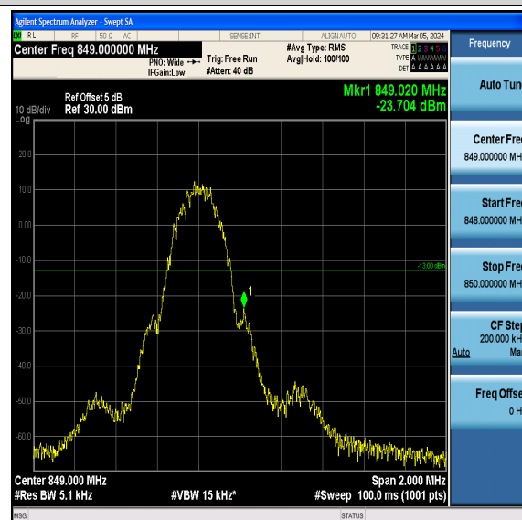
GPRS850-251
