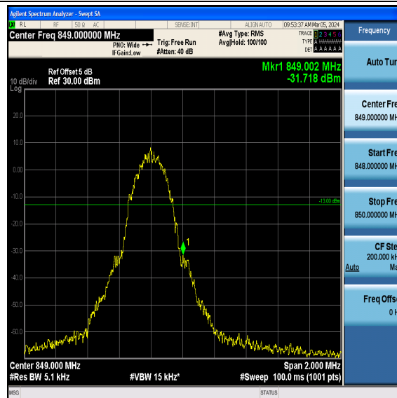
EGPRS850-251
