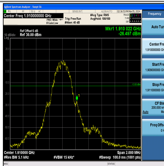
GPRS1900-810
