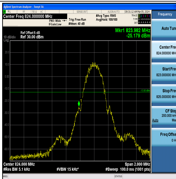
GPRS850-128
