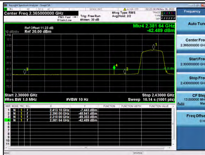
11G_Ant1_Low_2412_AV
