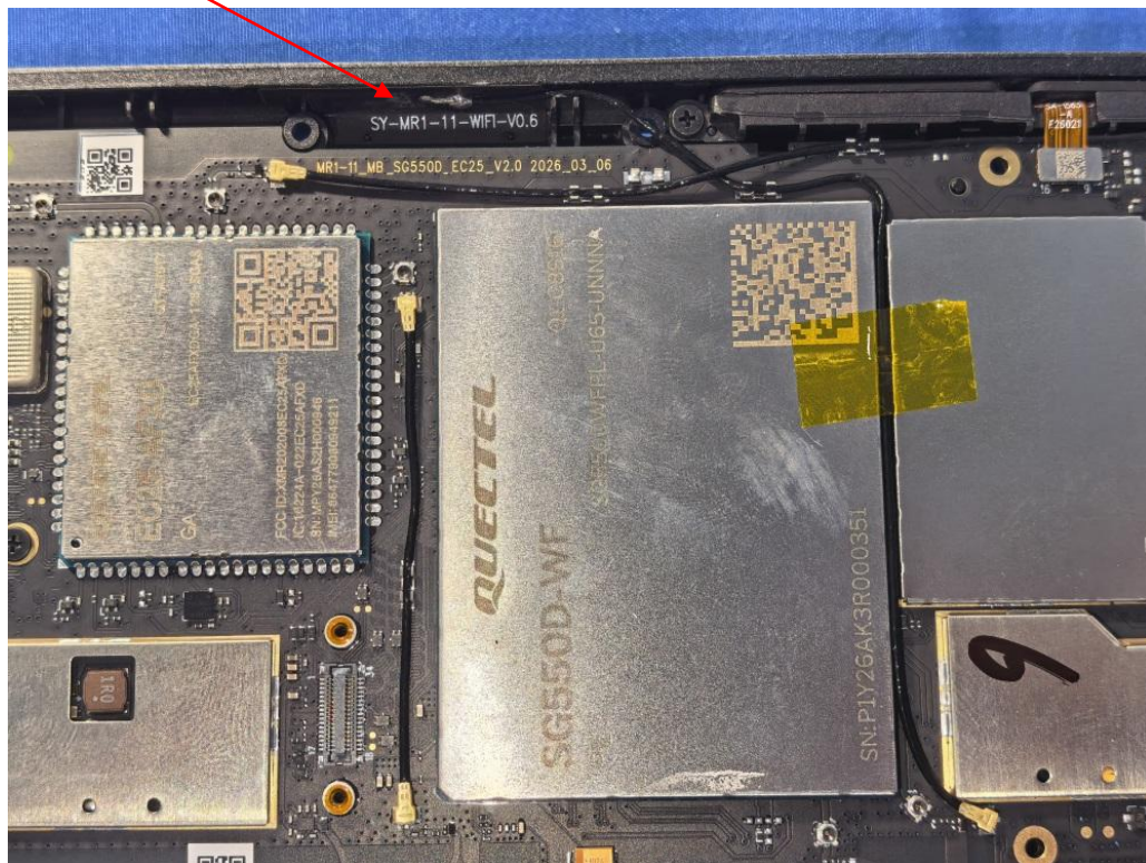
BT/WIFI Antenna 1
