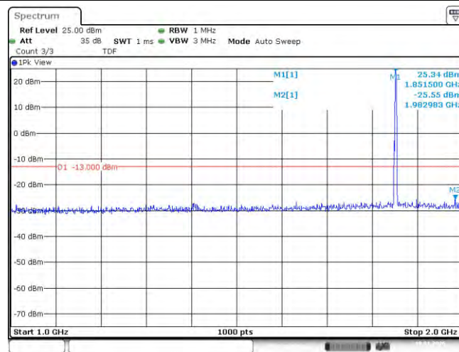
Band2-1.4MHz-QPSK-18607-6RB#0-Range2:1000~2000MHz
