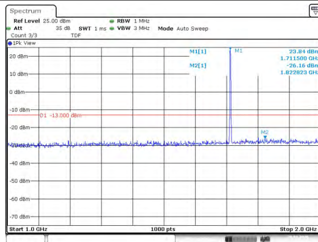
Band4-1.4MHz-QPSK-19957-6RB#0-Range2:1000~2000MHz
