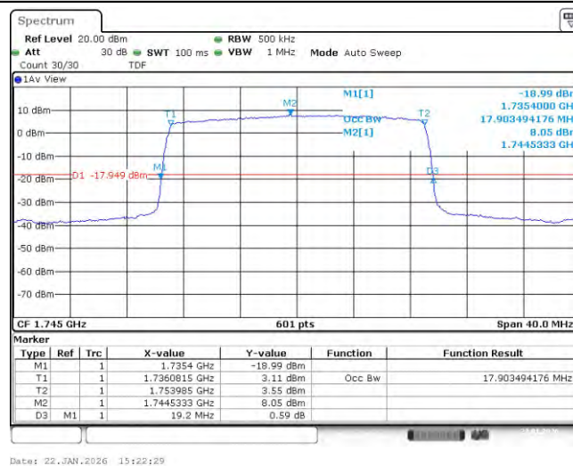
Band66-20MHz-QPSK-132572-100RB#0
