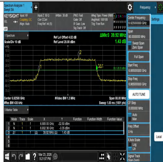
11ax40MIMO-Ant2-6925
