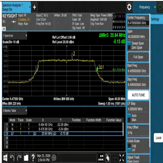
11ax20MIMO-Ant1-6475
