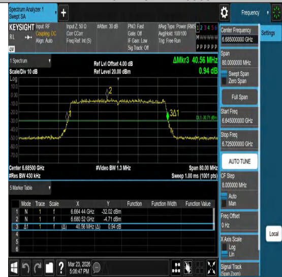
11ax40MIMO-Ant2-6685
