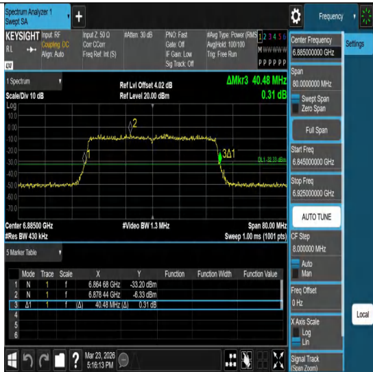
11ax40MIMO-Ant1-6885
