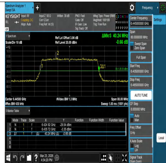
11ax40MIMO-Ant2-6445
