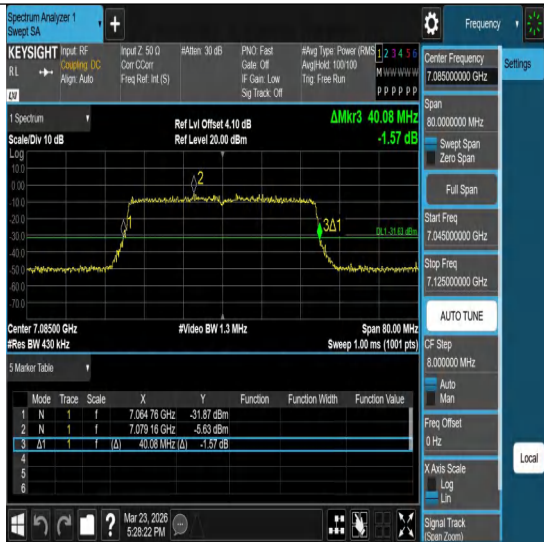
11ax40MIMO-Ant1-7085
