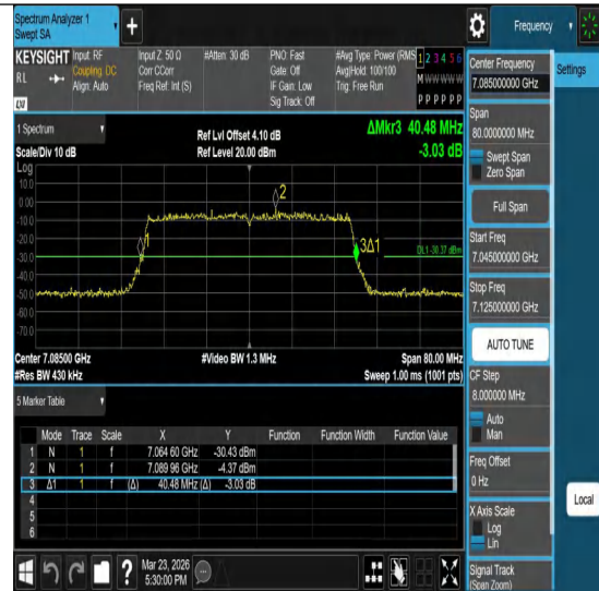
11ax40MIMO-Ant2-7085
