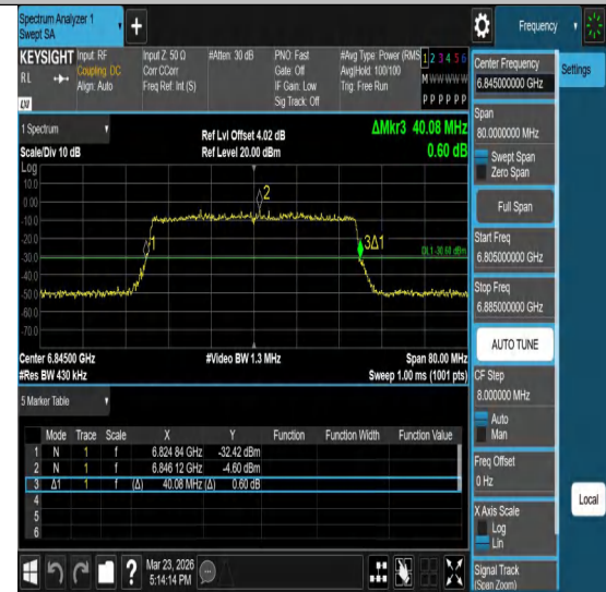
11ax40MIMO-Ant2-6845
