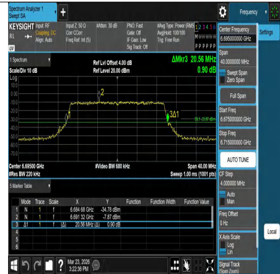
11ax20MIMO-Ant2-6695
