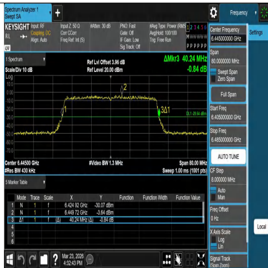
11ax40MIMO-Ant1-6445
