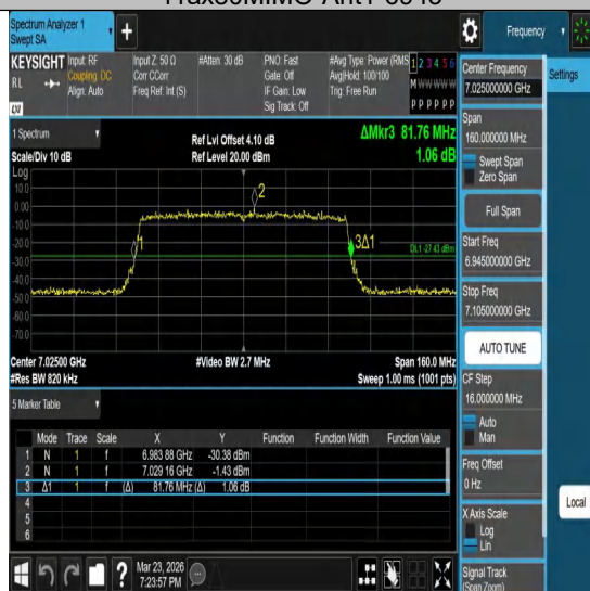
11ax80MIMO-Ant1-7025
