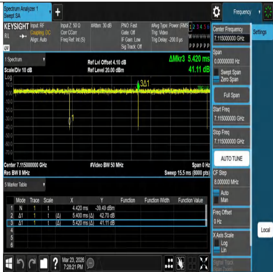
NTNV-11ac20MIMO-Ant1-7115
