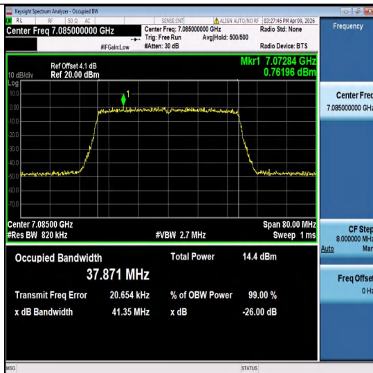
11ax40MIMO-Ant1-7085-PASS
