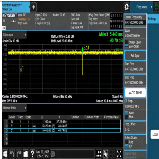
NTNV-11ax20MIMO-Ant1-6475
