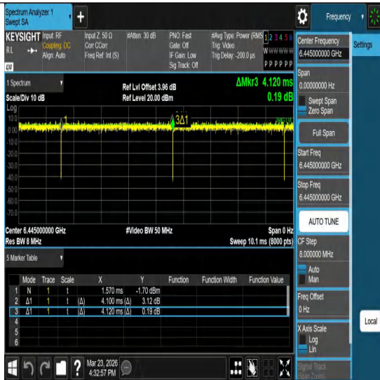
NTNV-11ax40MIMO-Ant1-6445
