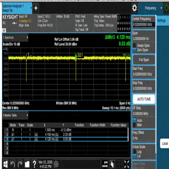
NTNV-11ax40MIMO-Ant1-6525
