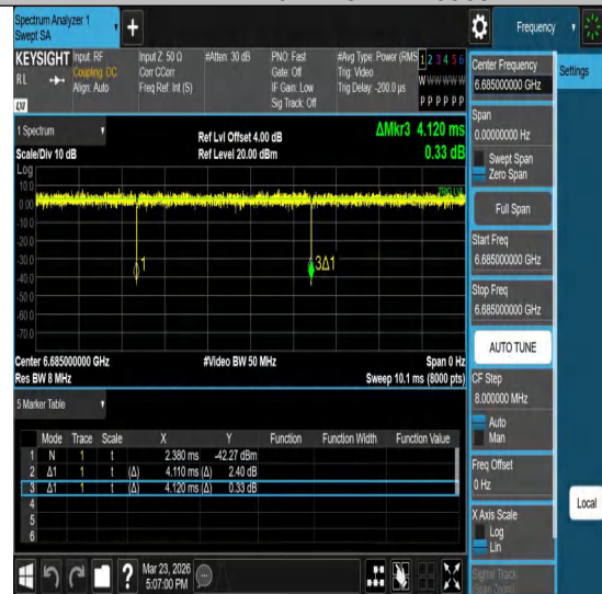
NTNV-11ax40MIMO-Ant2-6685
