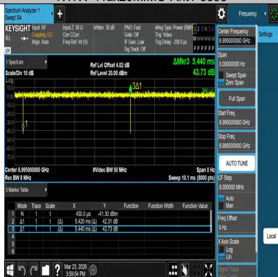
NTNV-11ax20MIMO-Ant1-6995
