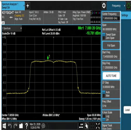
11ax40MIMO-Ant1-7085-PASS
