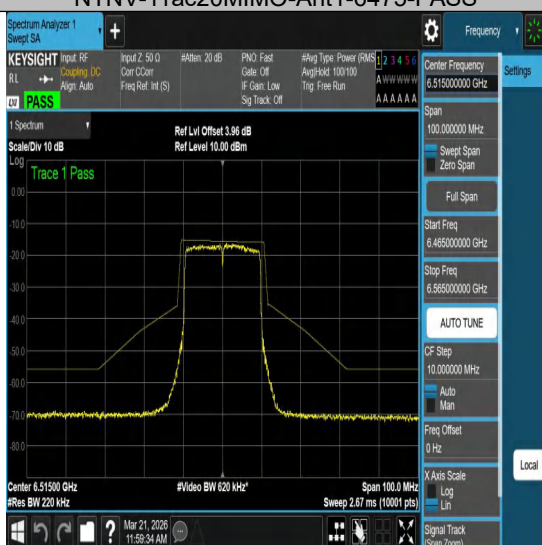
NTVN-11ac20MIMO-Ant1-6515-PASS
