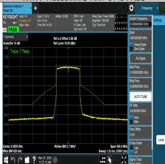
NTVN-11ac80MIMO-Ant1-6385-PASS
