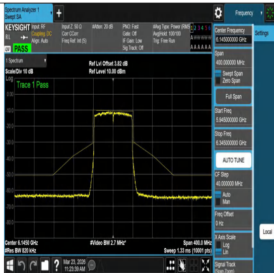
NTVN-11ac80MIMO-Ant1-6145-PASS
