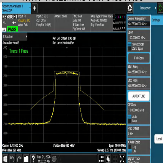
NTVN-11ac20MIMO-Ant1-6475-PASS
