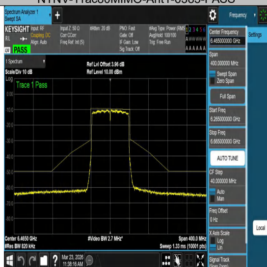
NTVN-11ac80MIMO-Ant1-6465-PASS
