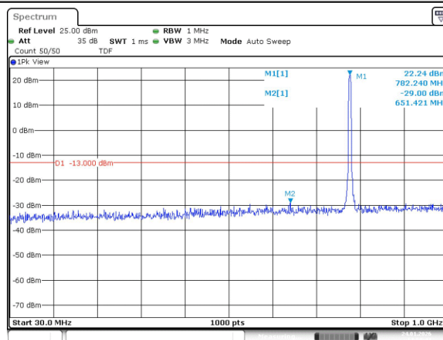
Band13-5MHz-QPSK-23230-25RB#0-Range1:30~1000MHz
