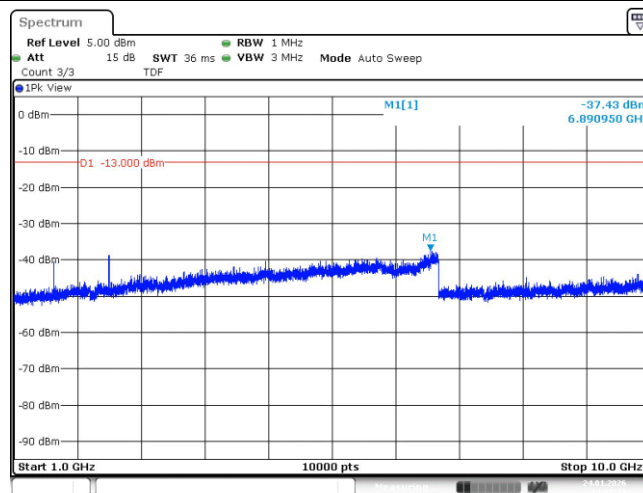
Band13-5MHz-QPSK-23205-25RB#0-Range2:1000~10000MHz
