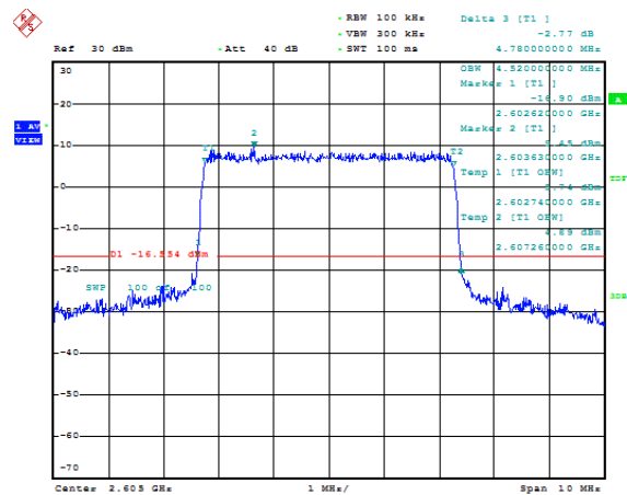
Band41-5MHz-QPSK-40740-25RB#0-4.52
