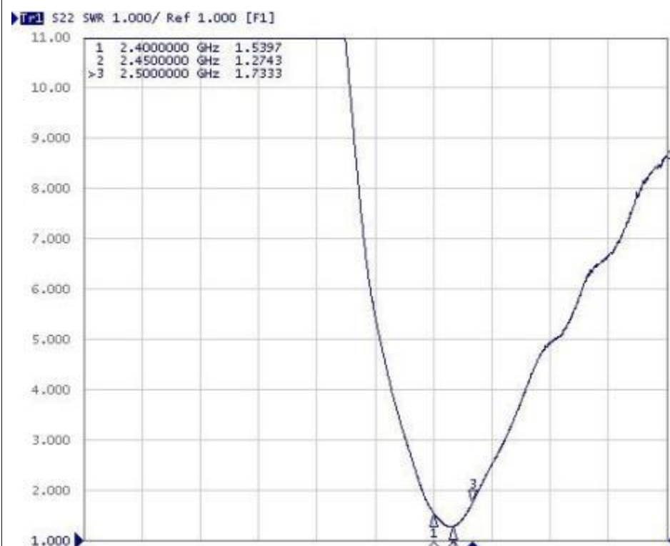
VSWR
