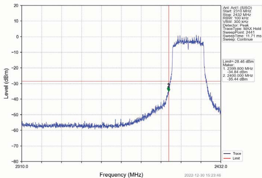
802.11ax(HEW20)_LCH_2412MHz_RU242_Left_Ant1 (SISO)_NTNV
