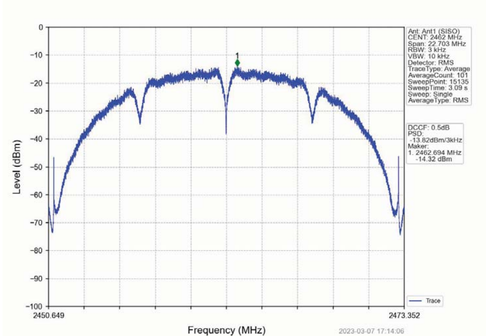
802.11b_HCH_2462MHz_Ant1 (SISO)_NTNV
