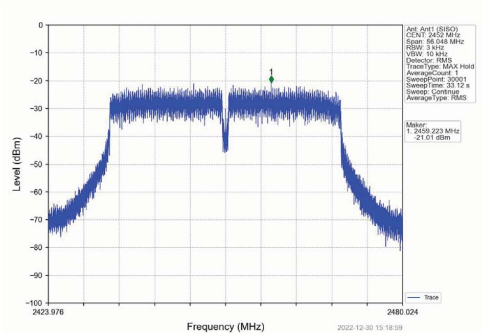
802.11n(HT40)_HCH_2452MHz_Ant1 (SISO)_NTNV
