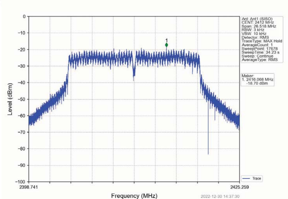
802.11g_LCH_2412MHz_Ant1 (SISO)_NTNV
