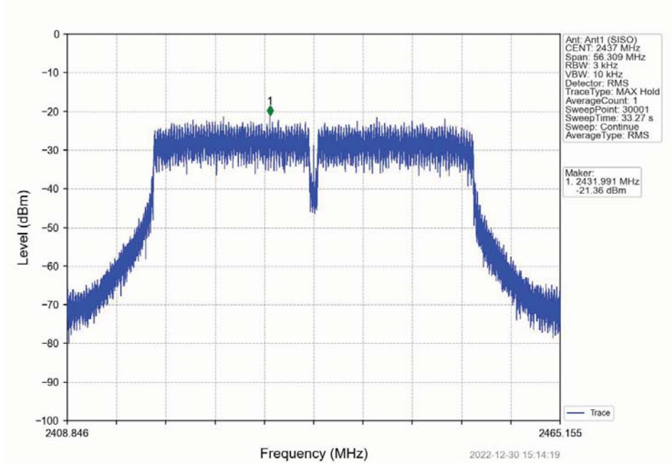
802.11n(HT40)_MCH_2437MHz_Ant1 (SISO)_NTNV
