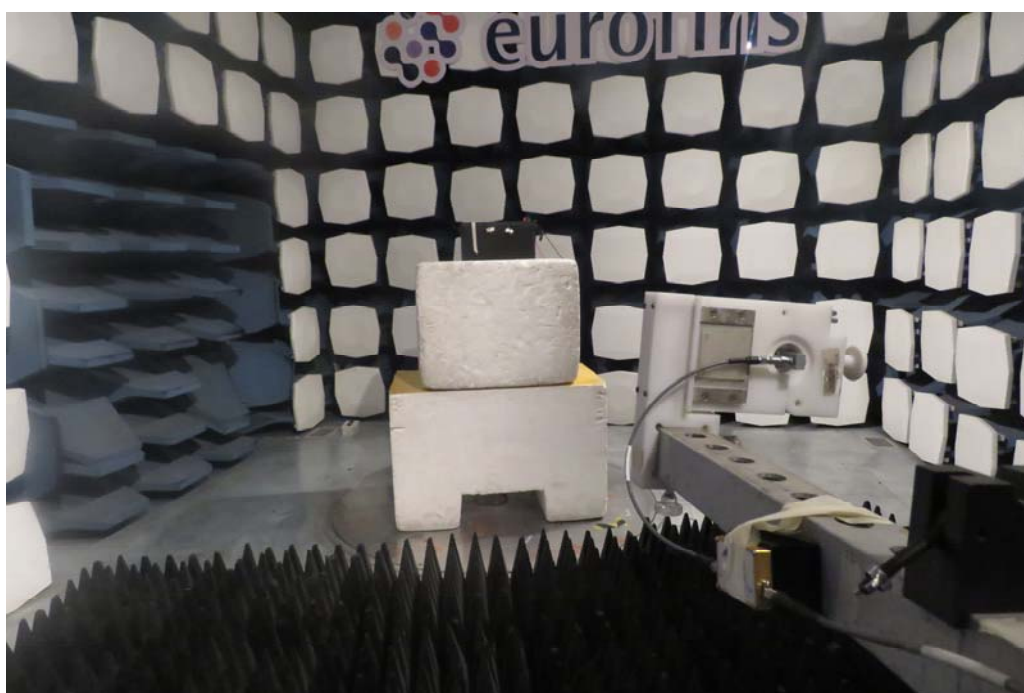
18GHz - 26.5GHz
